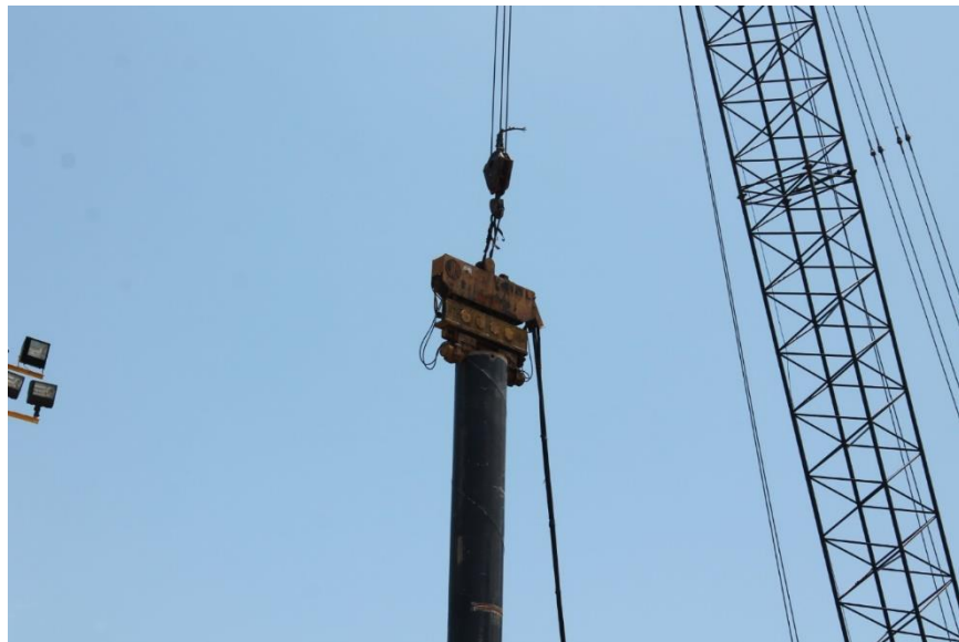
Figura 21. Hincado inicial con vibrador
