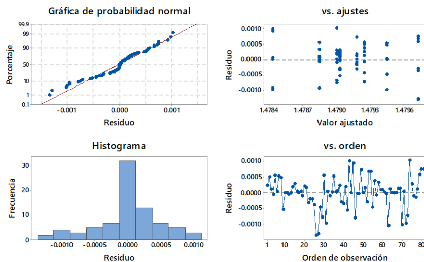
Figura 24. Gráficas de residuos para el índice de refracción a 20 °C del aceite esencial de la mandarina Dancy ( reticulata var. Dancy )
