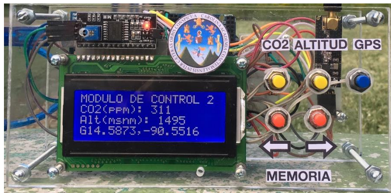
Figura 52. Módulo de control, banco de memoria 2
