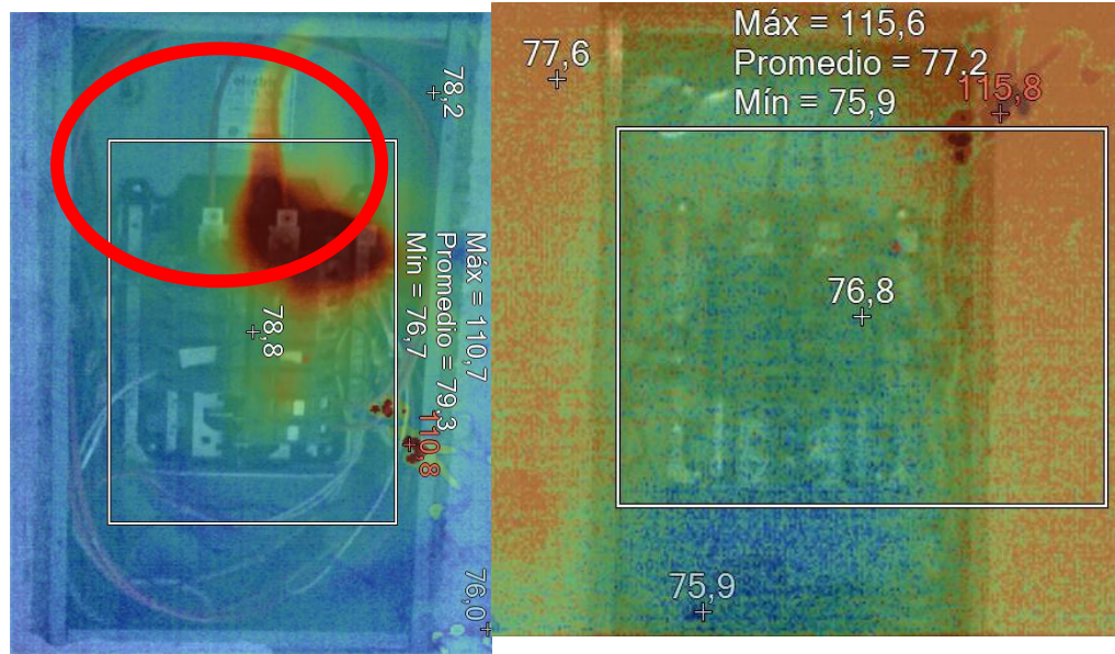
Figura 18. Fotografías tablero de distribución
