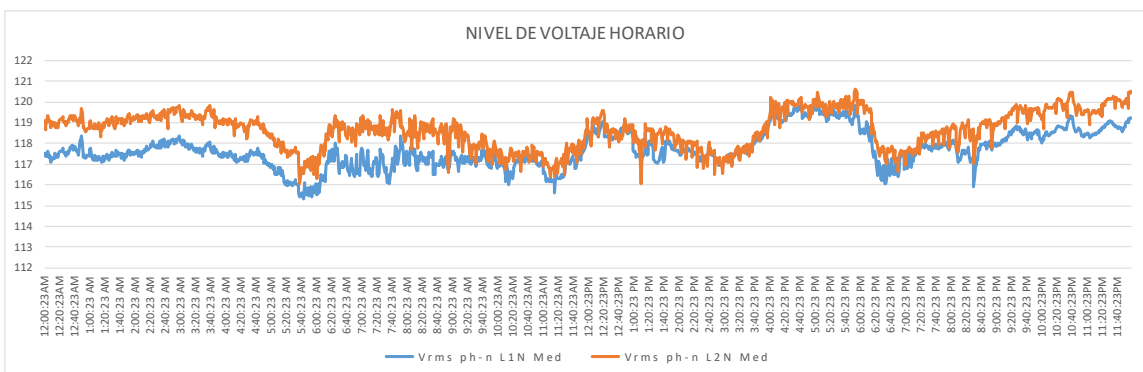
Figura 16. Niveles de voltaje horario
