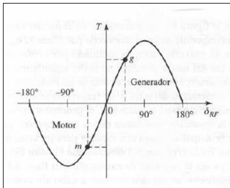
Figura 12. Gráfico del ángulo de par
