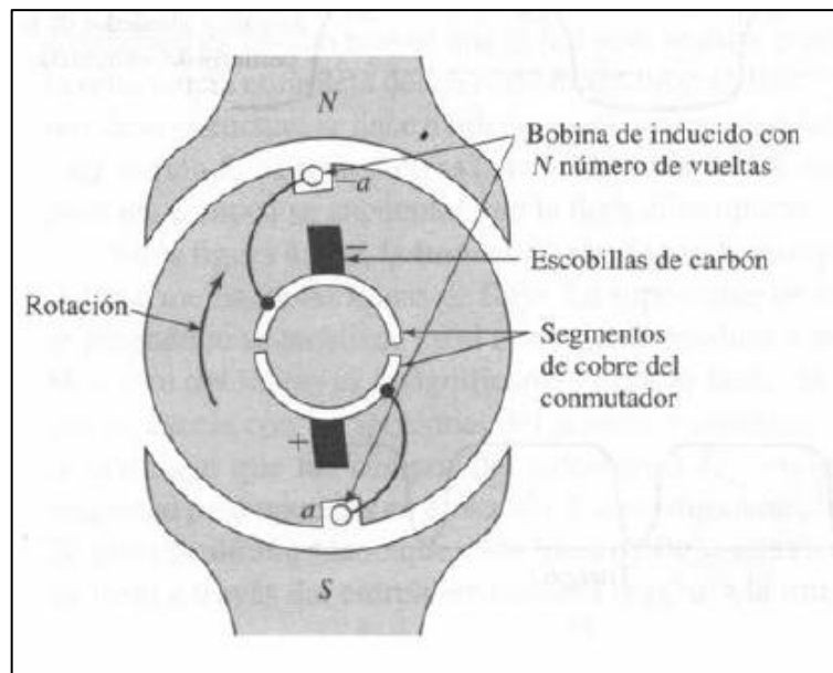
Figura 11. Máquina de corriente directa
