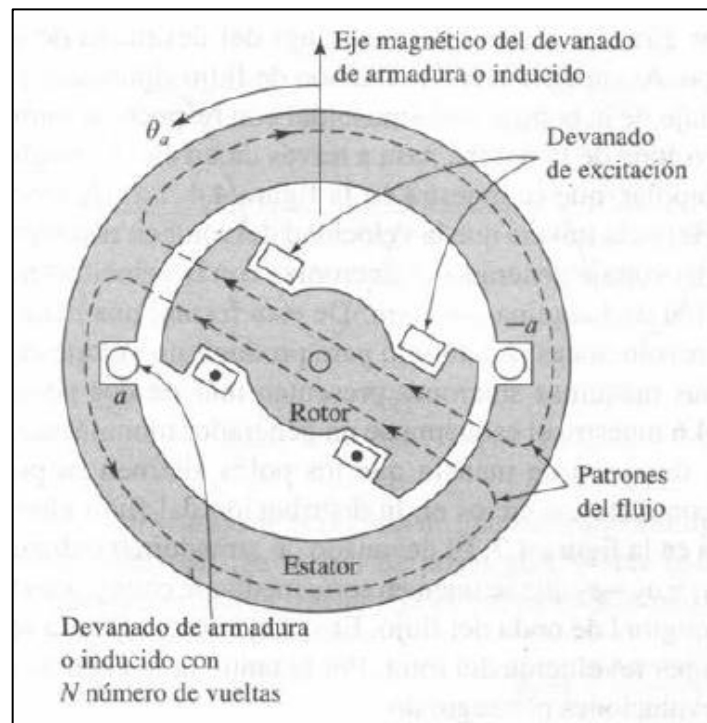
Figura 8. Generador síncrono de una fase y dos polos
