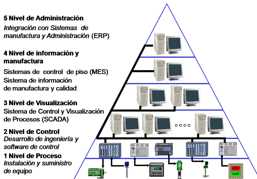
Figura 15. Pirámide de automatización
