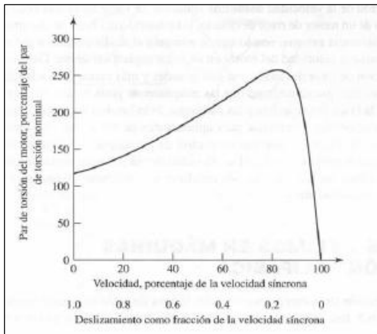
Figura 13. Curva par – velocidad del motor de inducción
