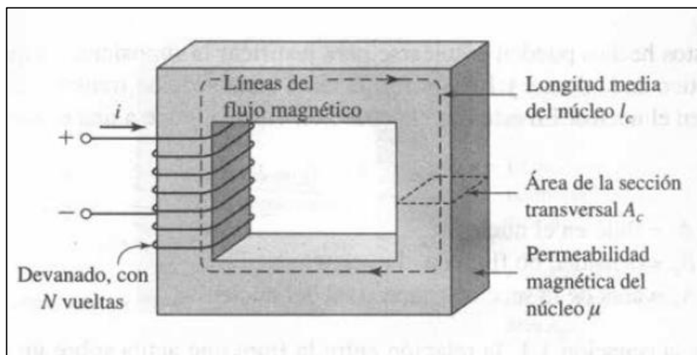
Figura 1. Circuito magnético simple
