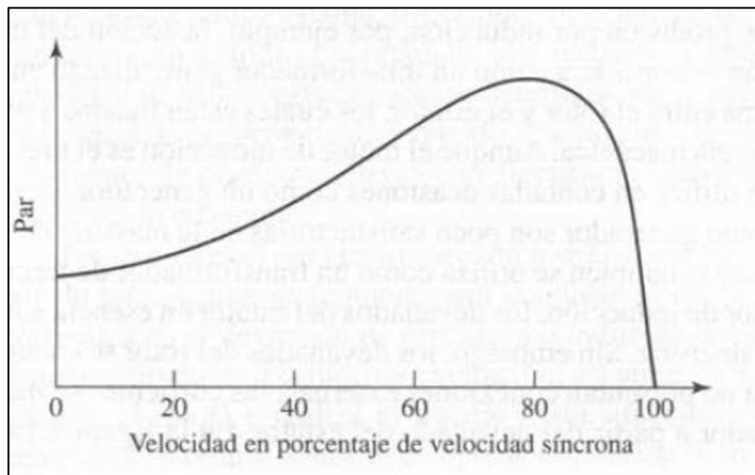
Figura 10. Características de velocidad y par de un motor de inducción
