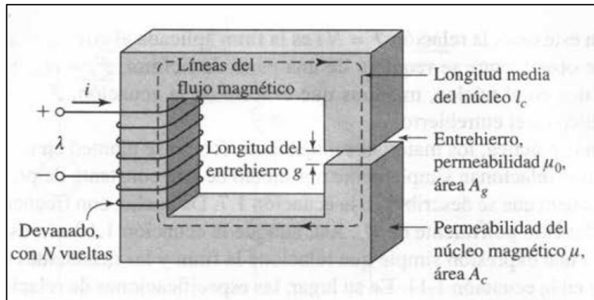
Figura 2. Circuito magnético con entrehierro
