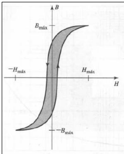
Figura 4. Curva de histéresis
