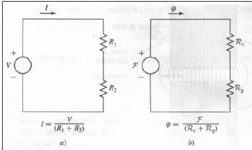
Figura 3. Relación circuito eléctrico y magnético
