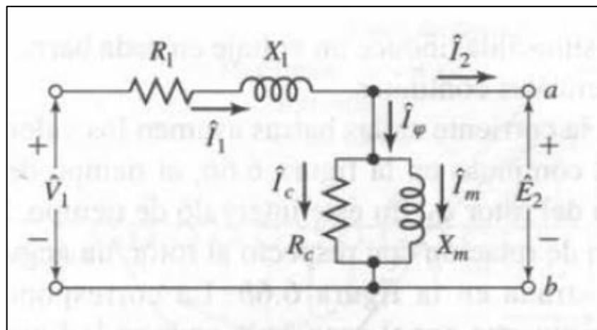
Figura 14. Circuito equivalente del motor de inducción polifásico
