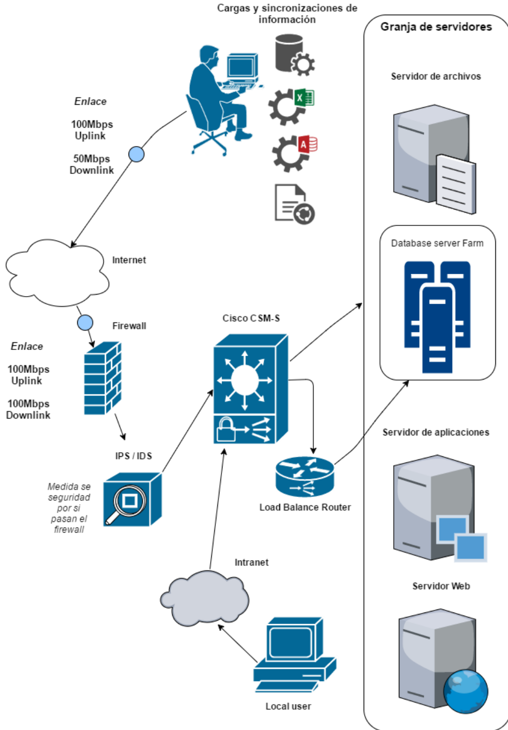
Figura 25. Esquema conceptual de la solución
