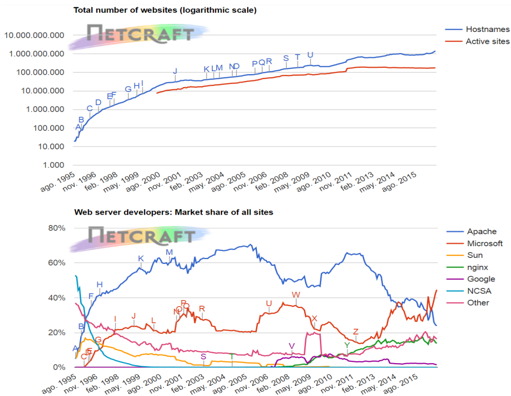
Figura 26. Rank de servidores web en el World Wide Web
