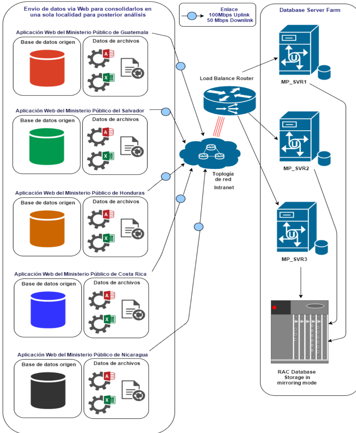
Figura 21. Modelo básico para consolidar información
