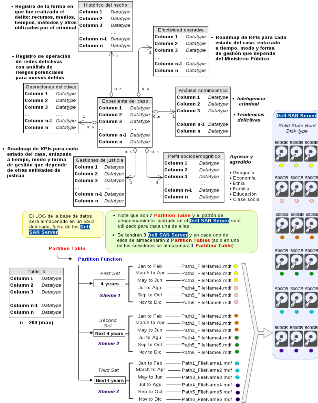
Figura 28. Modelo para gestionar base de datos e infraestructura
