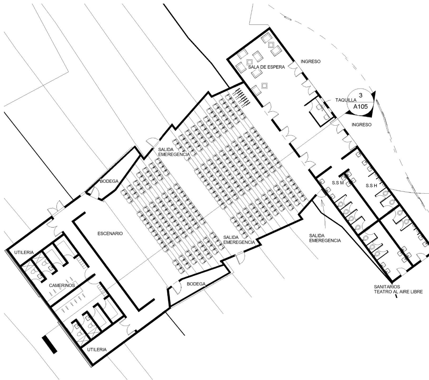
1 AUDITORIO 1 : 250
