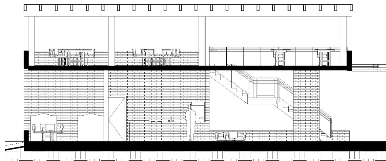
2 Sección 6 1 : 100
