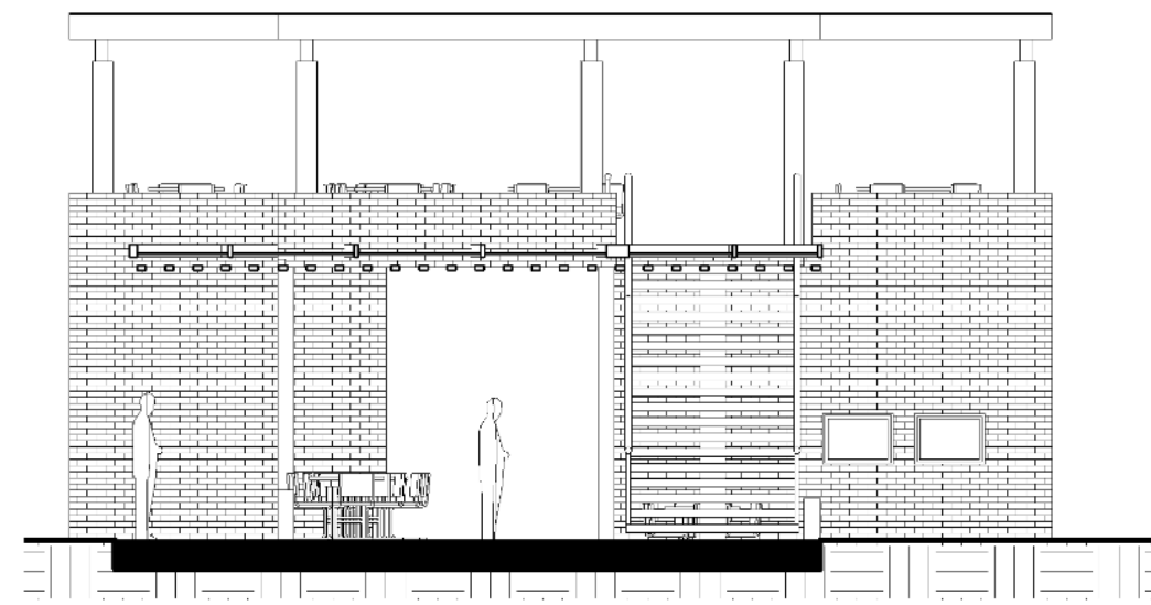
3 Alzado 1 : 100
