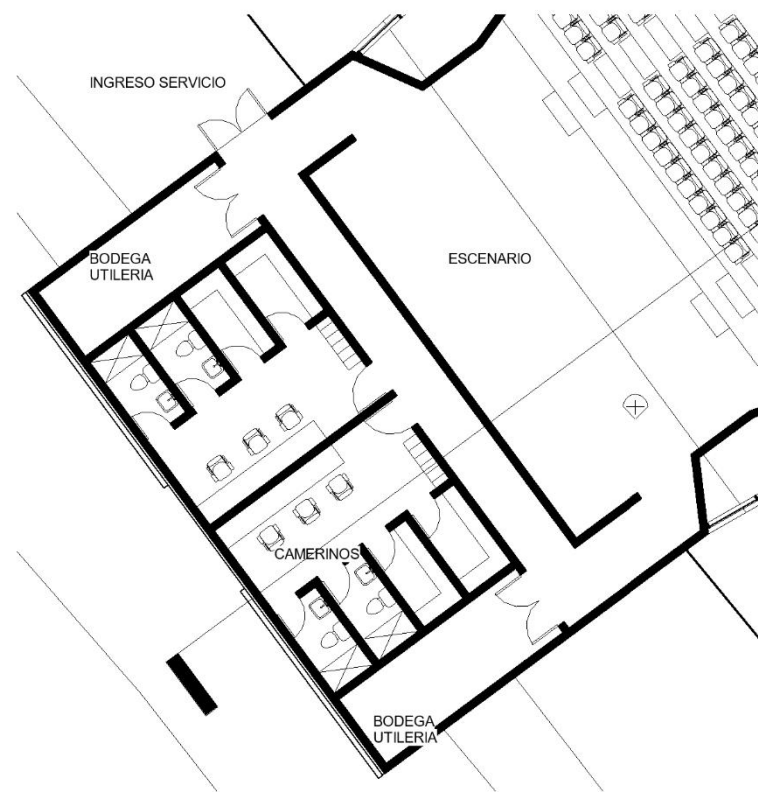
2 ESCENARIO 1 : 200
