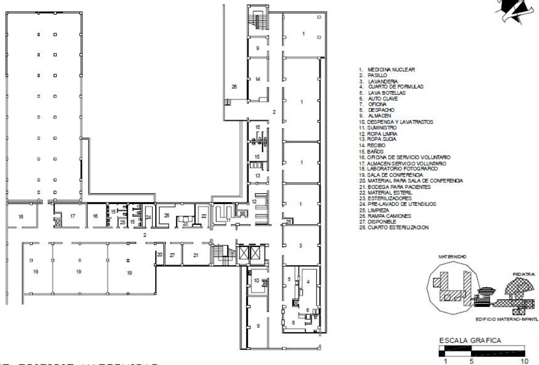
Figura 9: Planta de Sótano de Edificio de Maternidad
