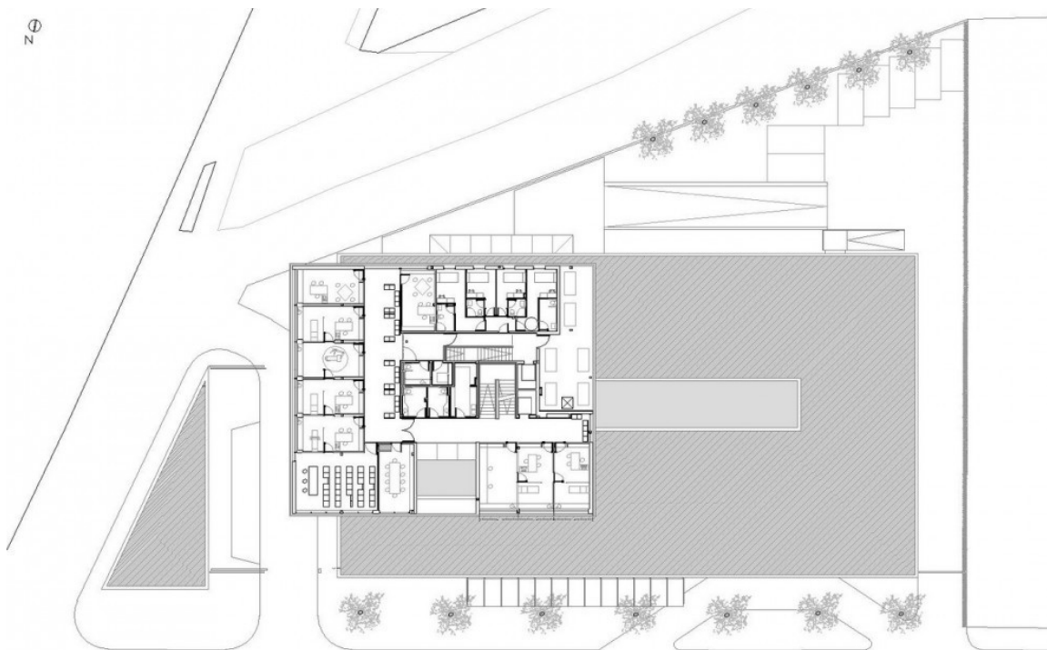
Figura 23: Planta de Segundo Nivel Fuente: www.hospitecna.com
