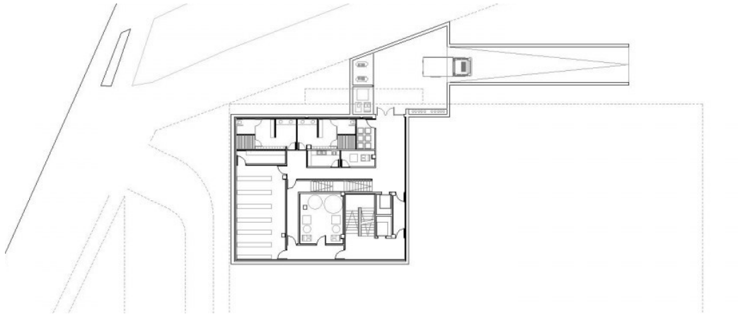
Figura 21: Planta de Sótano Fuente: www.hospitecnia.com
