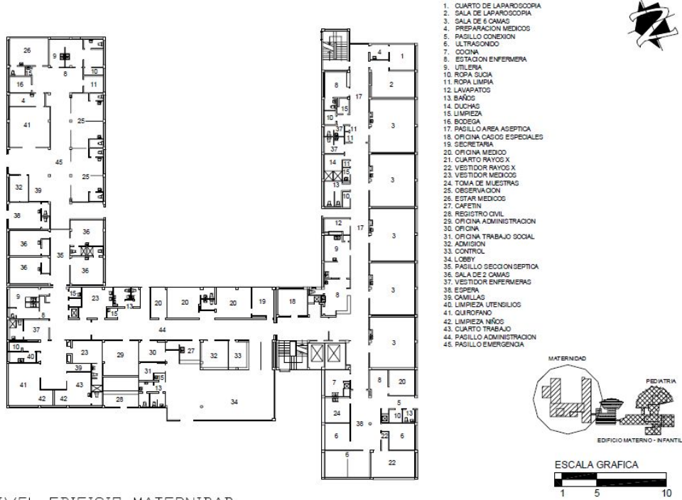
Figura 10: Planta de Primer Nivel de Edificio de Maternidad
