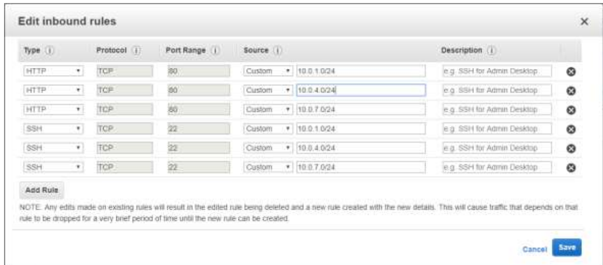
Figura 22. Configuración de firewall privado backend
