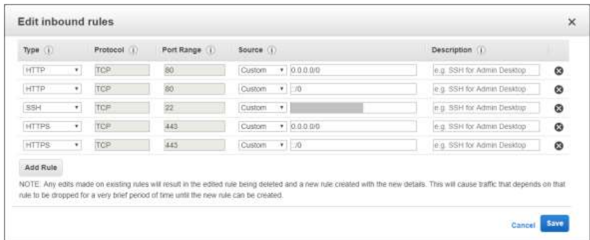
Figura 21. Configuración de firewall público
