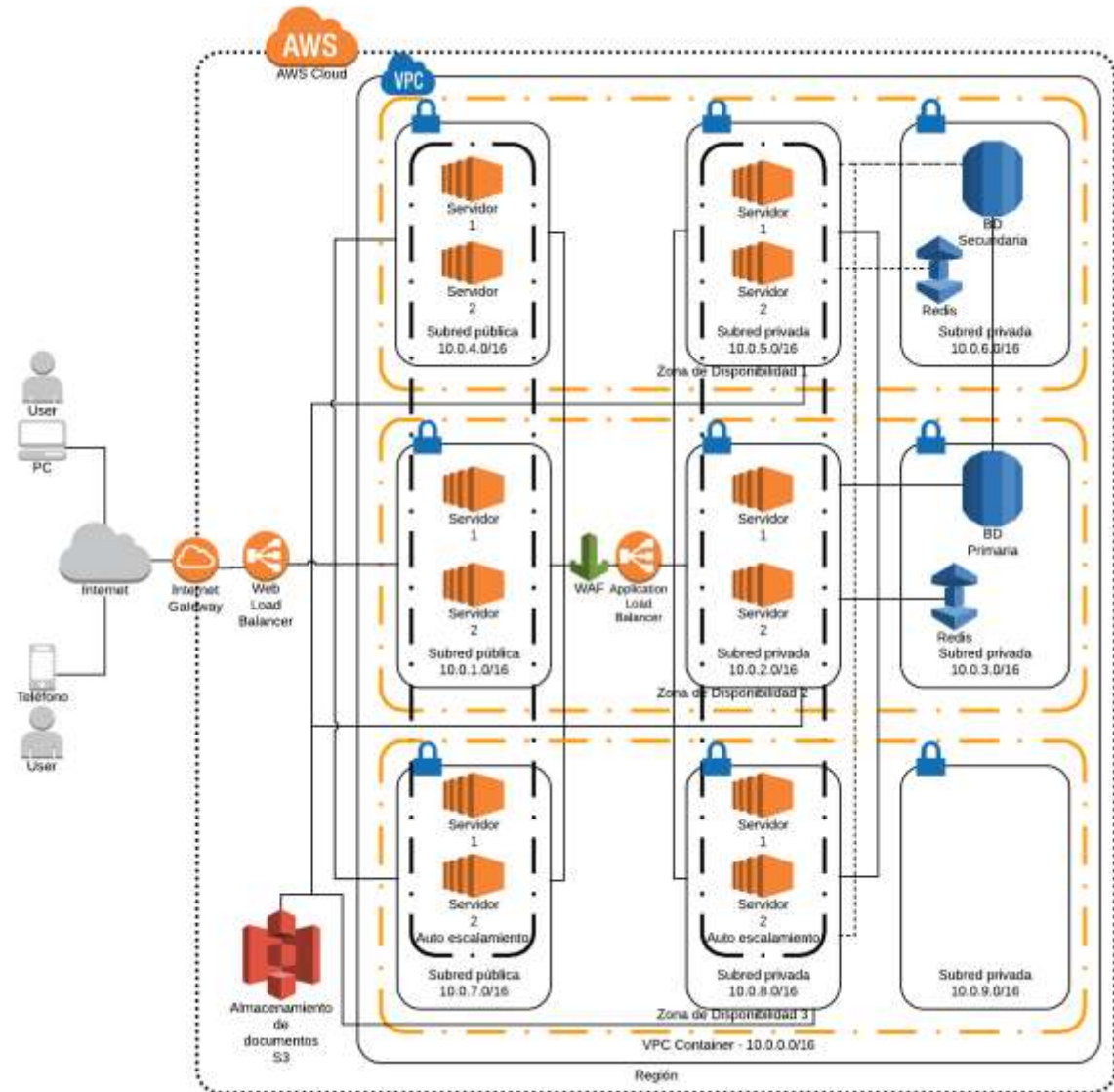
Figura 7. Arquitectura de solución
