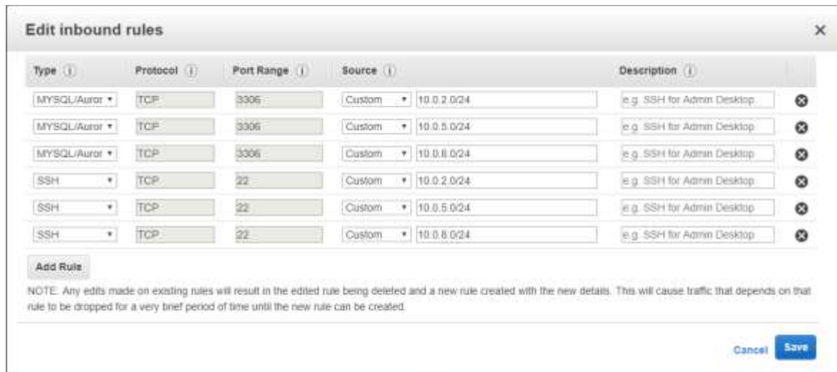
Figura 23. Configuración de firewall privado base de datos
