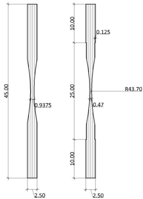
Figura 14. Probeta para ensayo de tensión paralelo a la fibra
