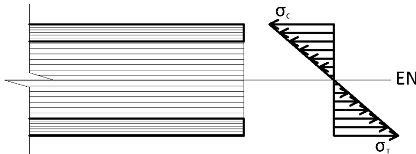
Figura 31. Distribución de esfuerzos por flexión
