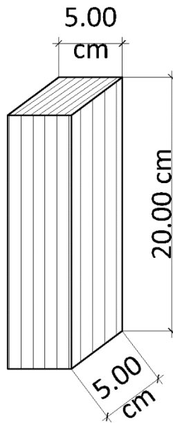
Figura 13. Probeta para ensayo de compresión paralelo a la fibra
