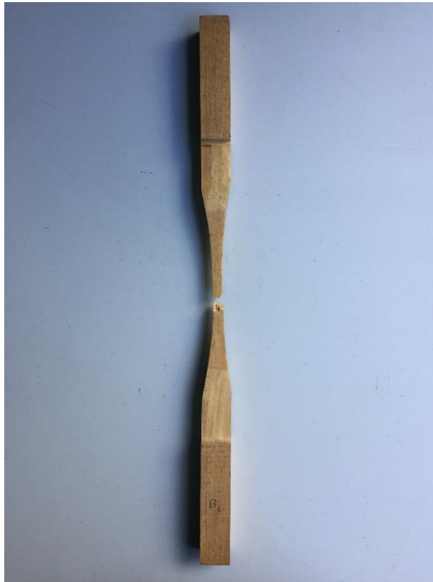
Figura 26. Probeta de tensión B2, falla por ruptura frágil
