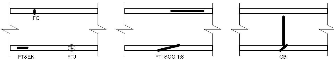
FIG. X5.2 Códigos de falla para puebas de escala completa
