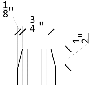
Figura 38. Detalle de canto de alma
