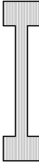
Figura 1. Sección típica, vigas tipo I
