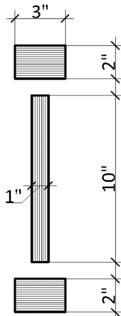
Figura 34. Pre dimensionamiento de vigas
