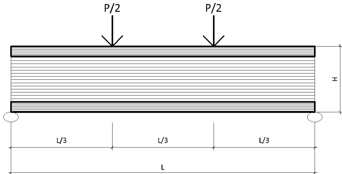
Figura 36. Esquema de ensayo a flexión en viga I
