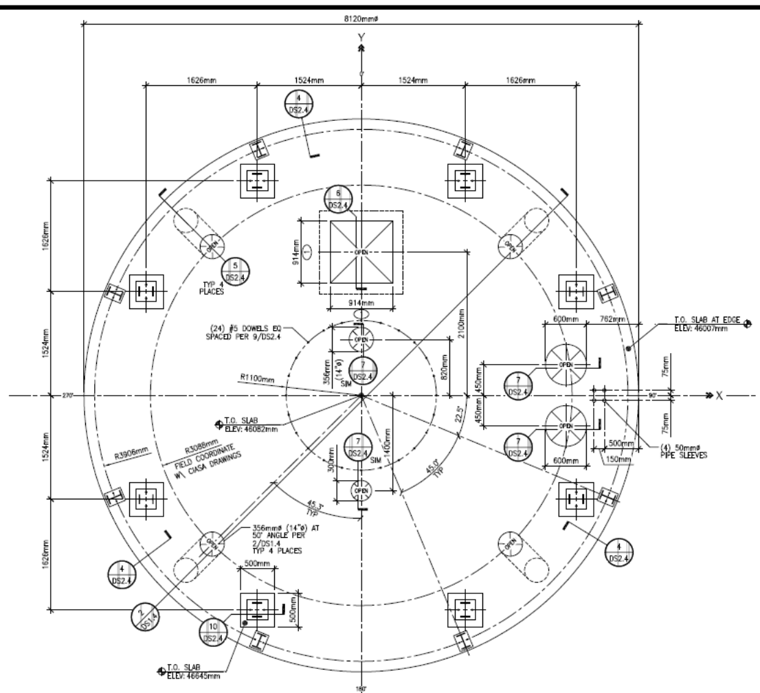
Planta de Losa de Apex
