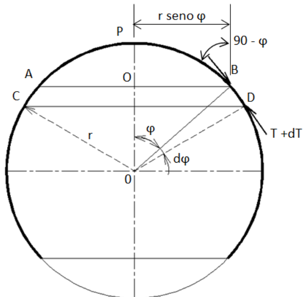
Figura 10. Sección de domo esférico
