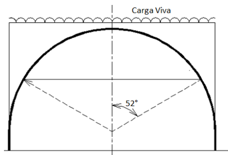
Figura 13. Distribución de carga viva
