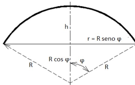
Figura 12. Datos de geometría de domo
