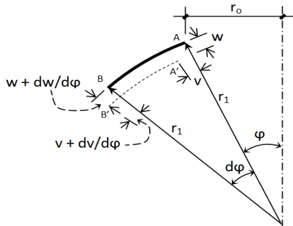
Figura 3. Desplazamientos en el elemento de cascarón
