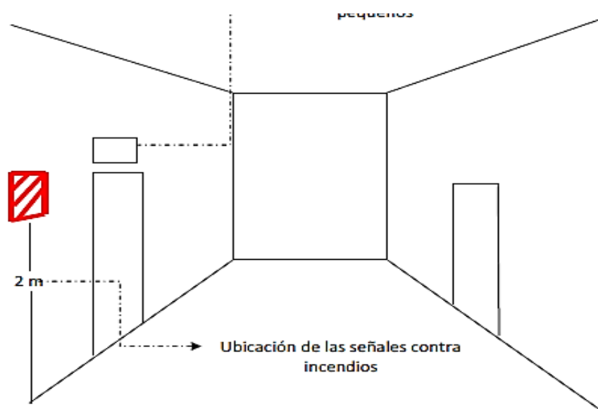
Figura 31. Ubicación del rótulo de señalización de extintores
