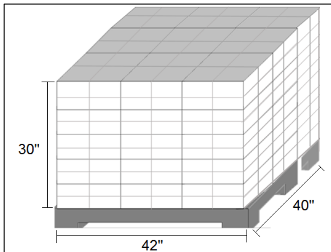
Figura 17. Entarimado 2, para 420 ejemplares de 6"x6" (42 ejemplares en base y 10 hacia arriba)
