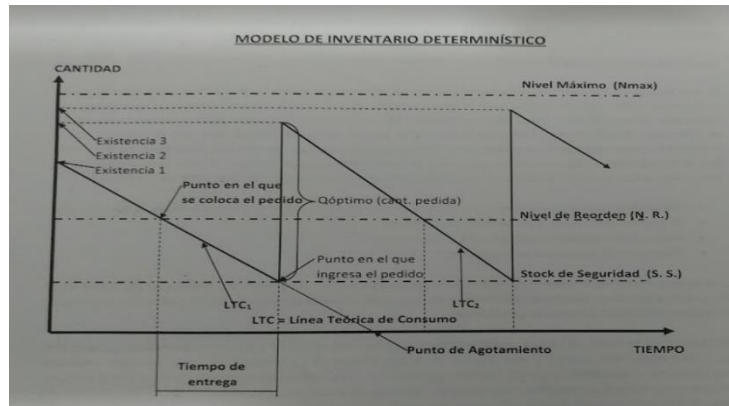
Figura 44. Modelo de inventario determinístico
