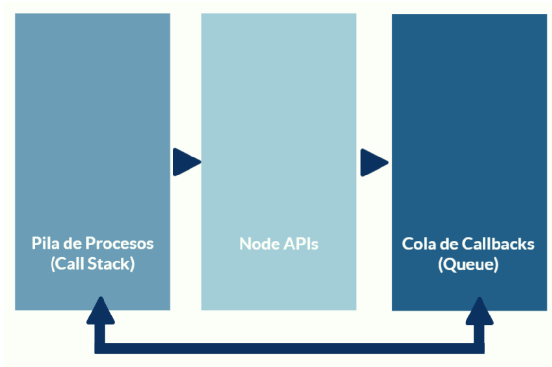
Figura 69. Ciclo de vida de un proceso en Node.js
