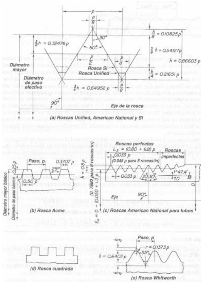
Figura 26. Tipos de roscas
