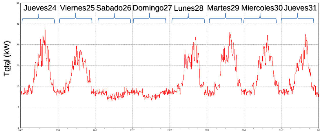
Figura 18. Curva de carga semanal total, valores máximos (kW)
