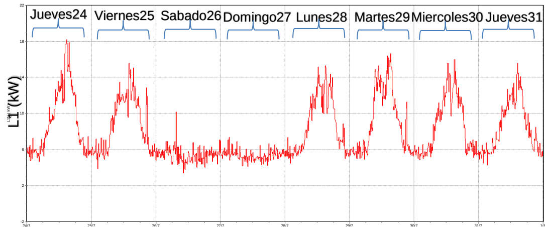
Figura 19. Curva de potencia semanal línea 1, valores máximos
