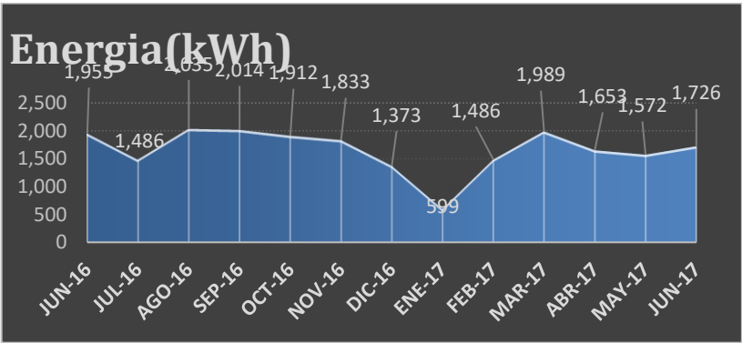
Figura 29. Área energía vs. periodo
