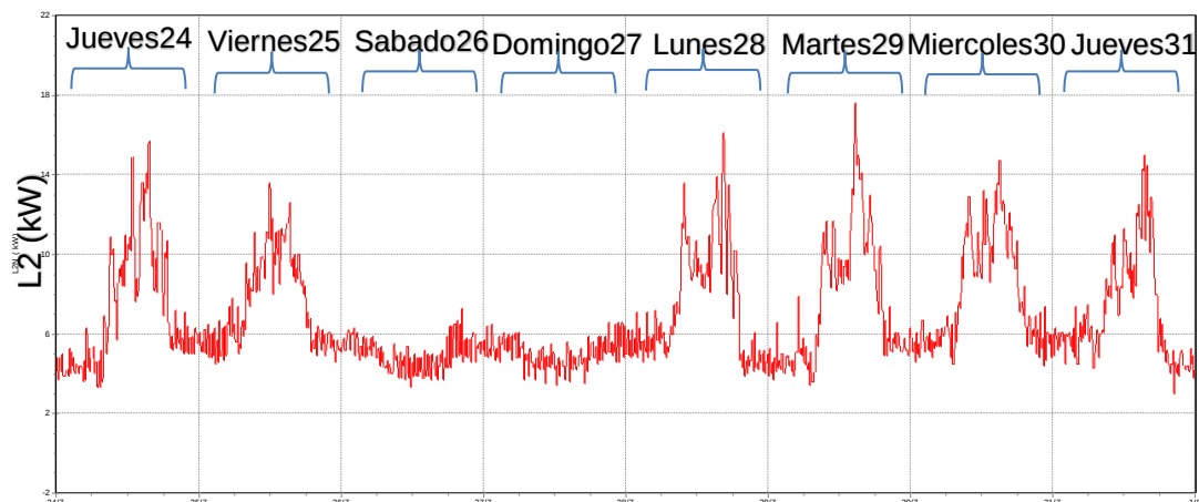
Figura 20. Curva de potencia semanal línea 2, valores máximos
