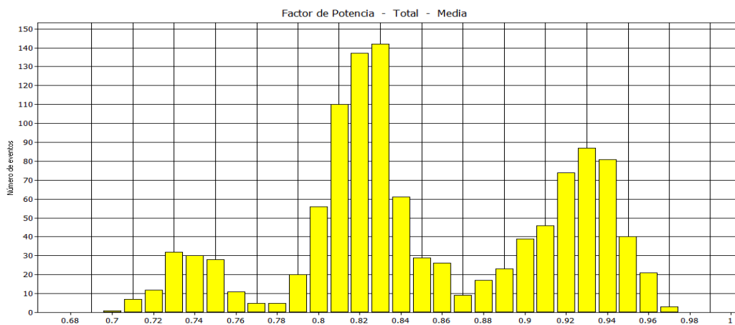
Figura 23. Estadística de factor de potencia total
