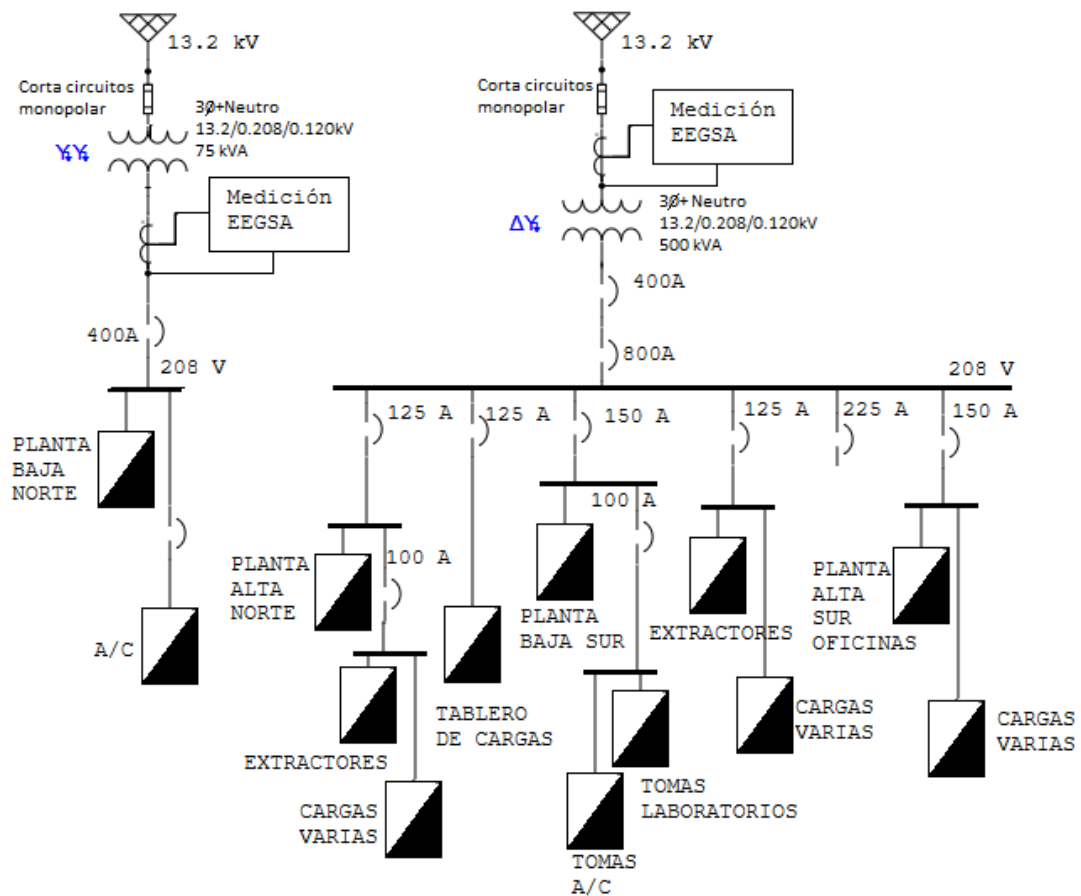
Figura 8. Diagrama unifilar eléctrico del edificio T-12, zona 12 campus central, Universidad de San Carlos de Guatemala
