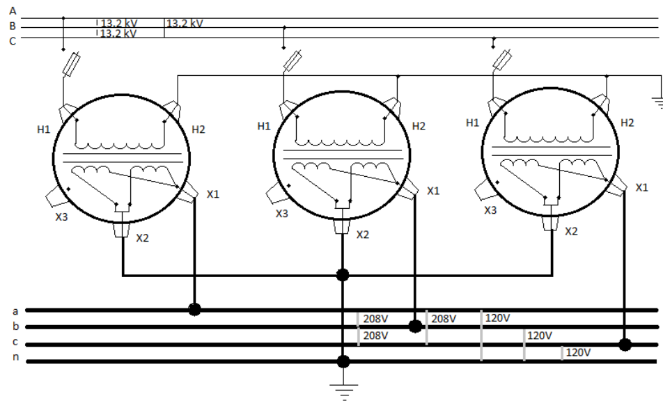
Figura 11. Diagrama de conexión del banco de transformadores conexión Y-Y aterrizado, cuatro hilos
