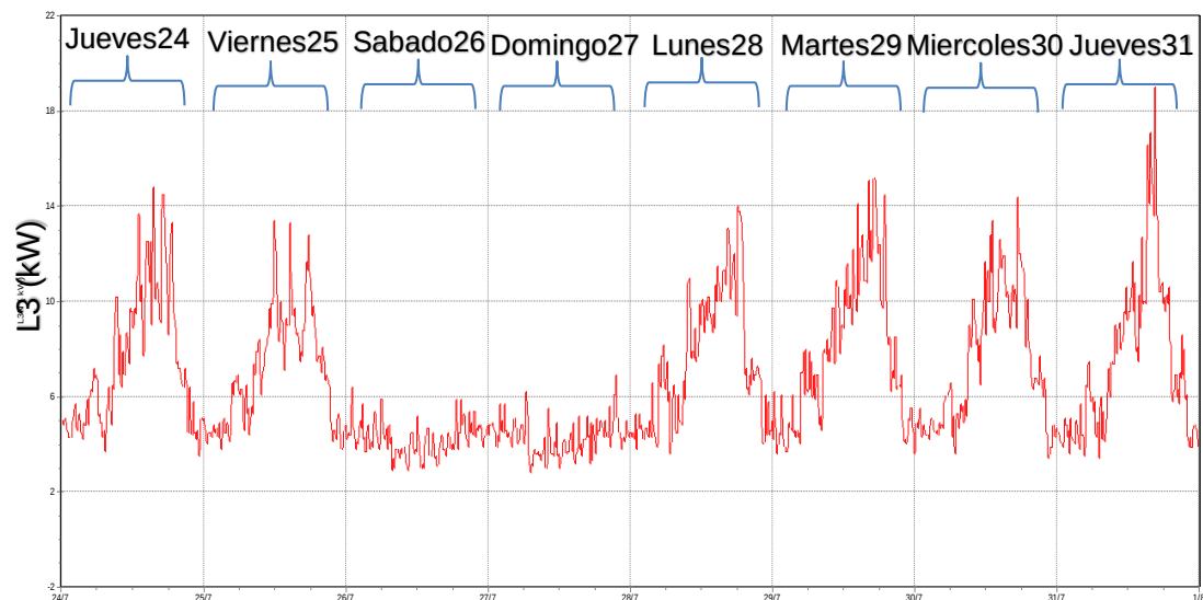
Figura 21. Curva de potencia semanal línea 3, valores máximos
