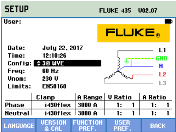
Figura 14. Configuración tipo: trifásica estrella (Y) aterrizada (3Ø WYE)
