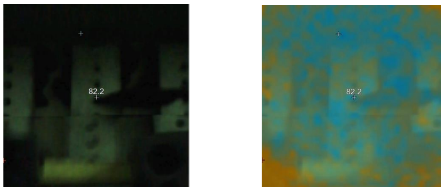
Figura 35. Temperatura en barras, tablero principal
