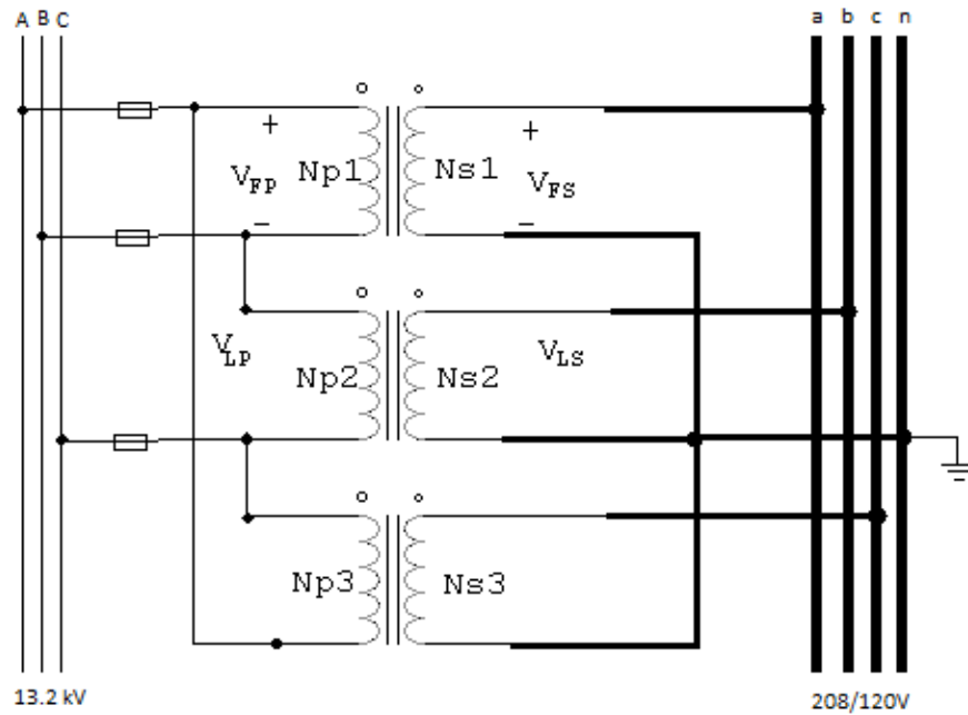
Figura 9. Diagrama de conexión del transformador tipo pad-mounted conexión \Delta -Y aterrizado, cuatro hilos
