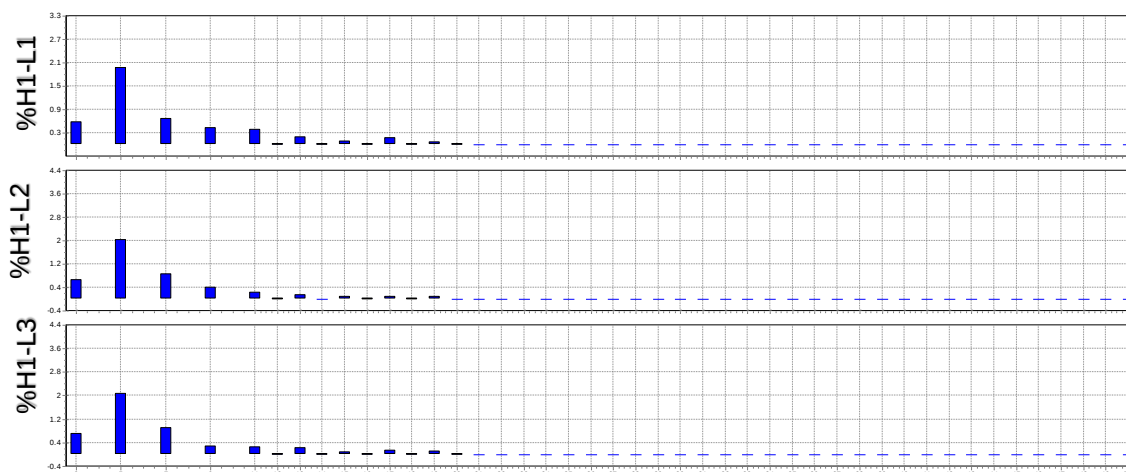
Figura 24. Representación hasta el 50 armónico de la L1, L2, L3
