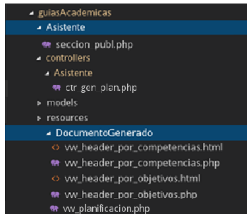
Figura 117. Estructura para planificación
