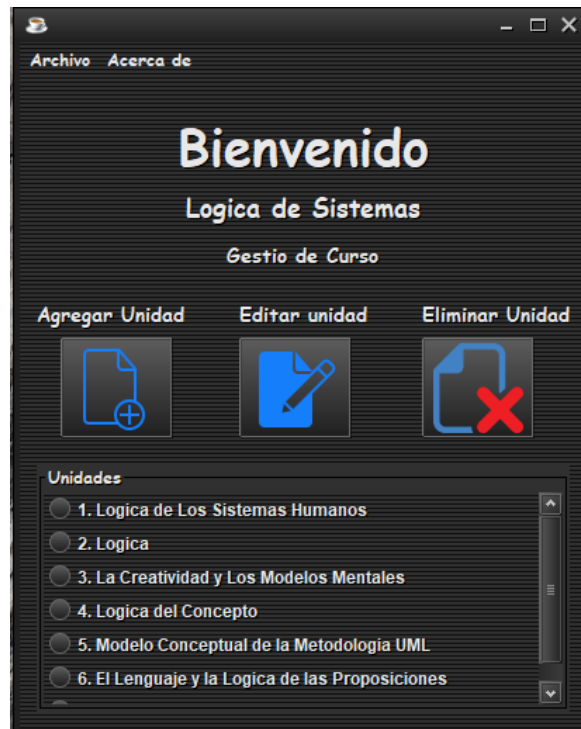
Figura 10. Módulo administrador – gestión de curso
