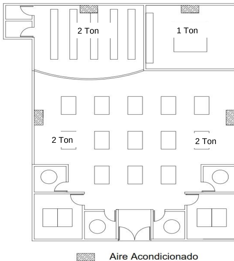
Figura 16. Plano de distribución del sistema de ventilación de la EFPEM
