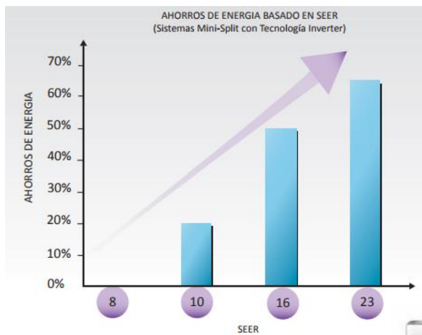
Figura 13. Ahorros de energía basados en sistemas Inverter
