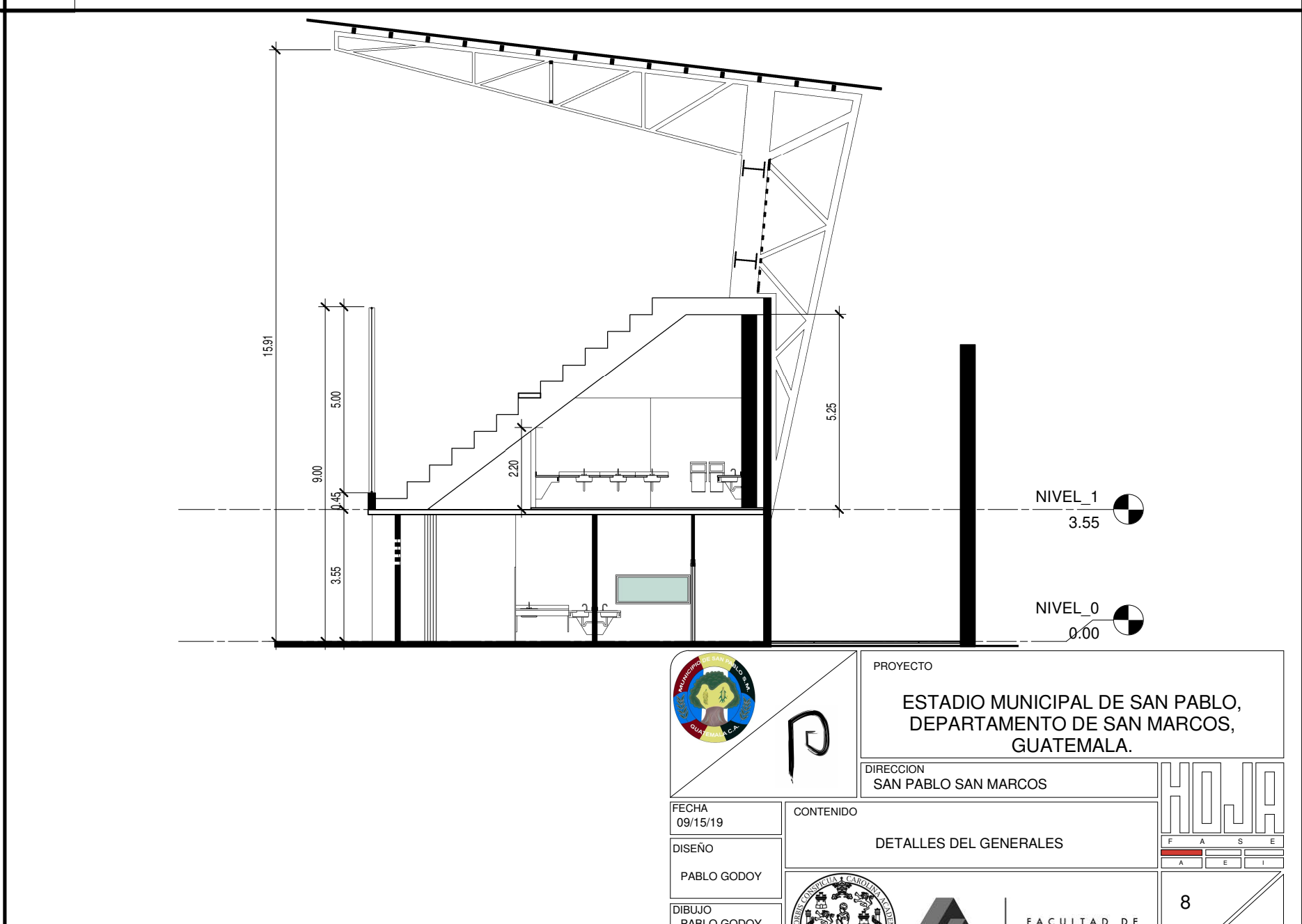
A10 DETALLE DE GRADERIOS ESC. 1 : 100
