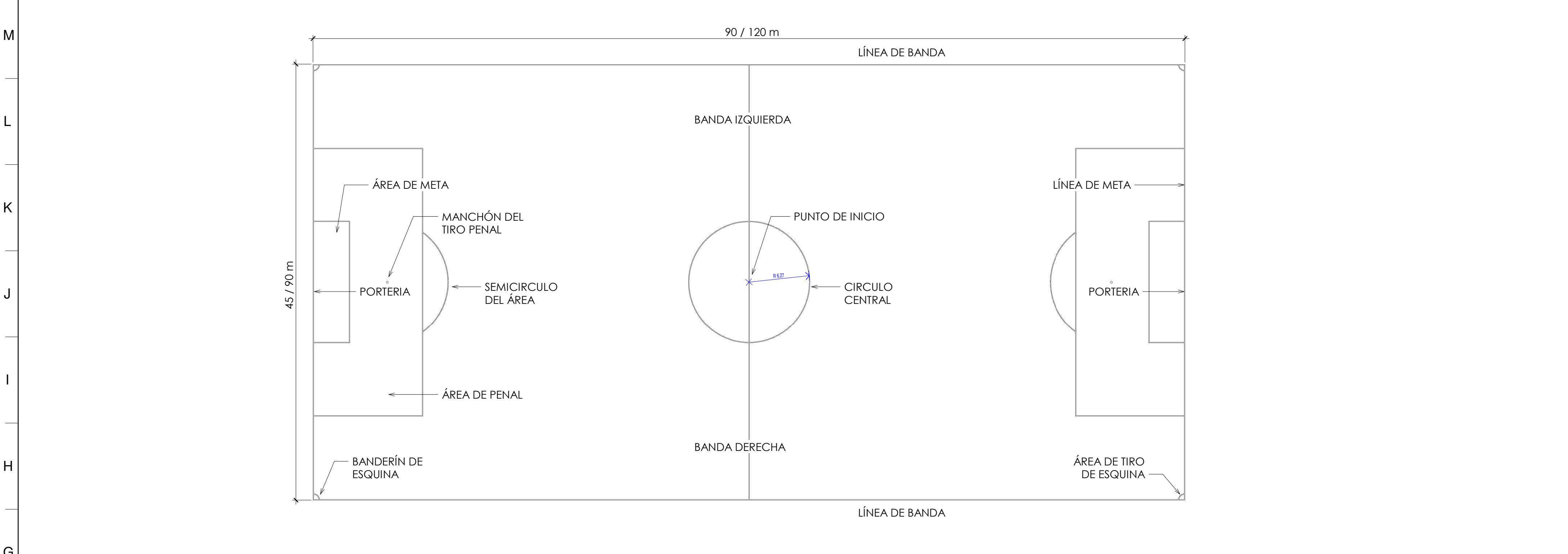
G1 DETALLE DE PARTES Y DIMENSIONES DE TERRENO DE JUEGO ESC. 1 : 200
