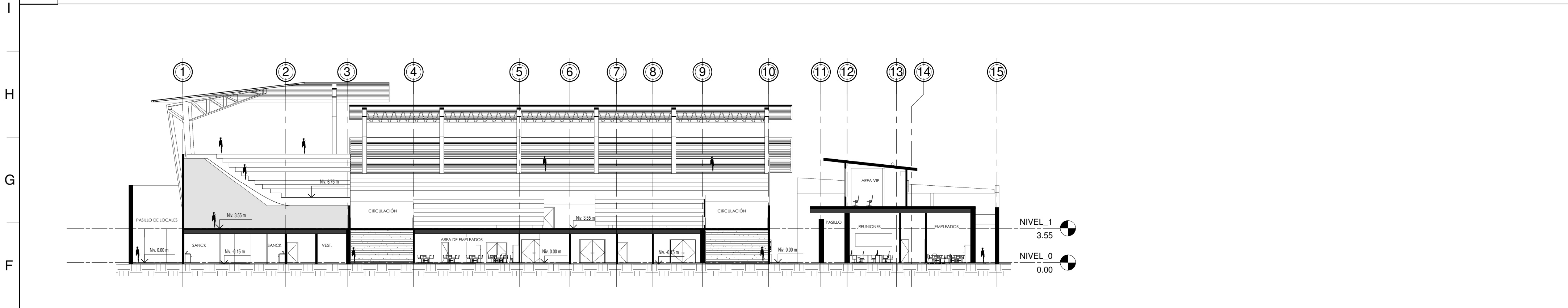
E1 SECCION B-B ESC. 1 : 200
