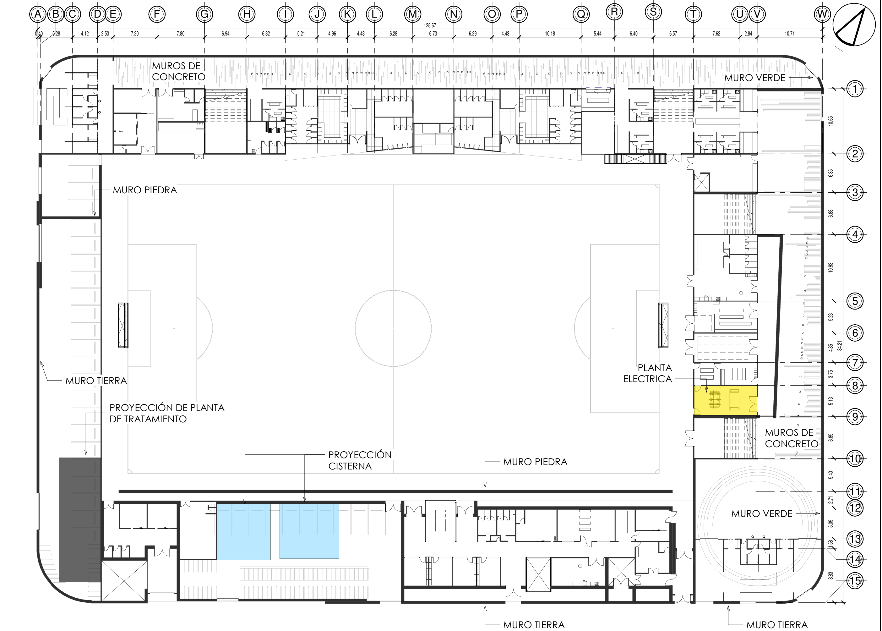
D6 INSTALACIONES ESC. 1 : 275
