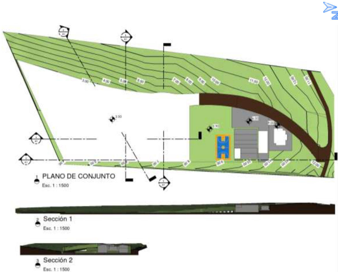
Figura 67, Plano topográfico y secciones del conjunto. Elaboración propia, Guatemala, febrero 2019
