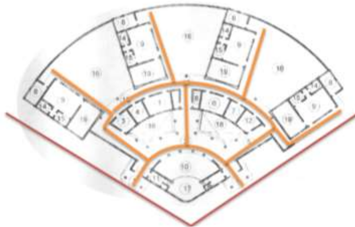
Figura 23, Planta del conjunto de la Escuela Tipo Federación http://biblioteca.usac.edu.gt/tesis/02/02_1622.pdf
