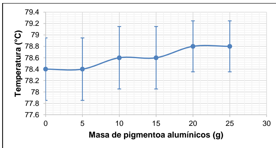
Figura 5. Ascenso de la temperatura de ebullición para el solvente etanol
