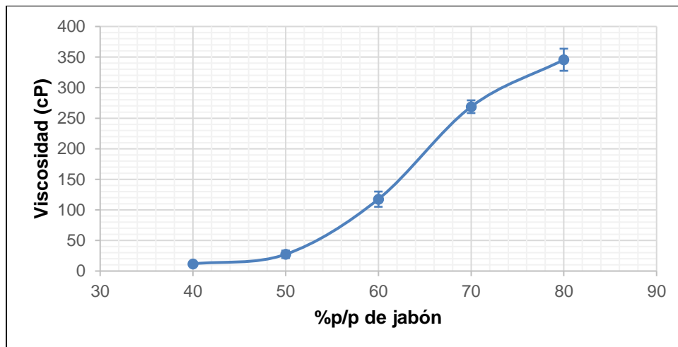
Figura 6. Viscosidad de la mezcla en función del porcentaje en peso del jabón en acetona
