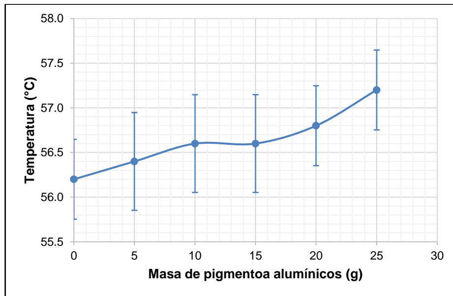
Figura 3. Ascenso de la temperatura de ebullición para la solvente acetona
