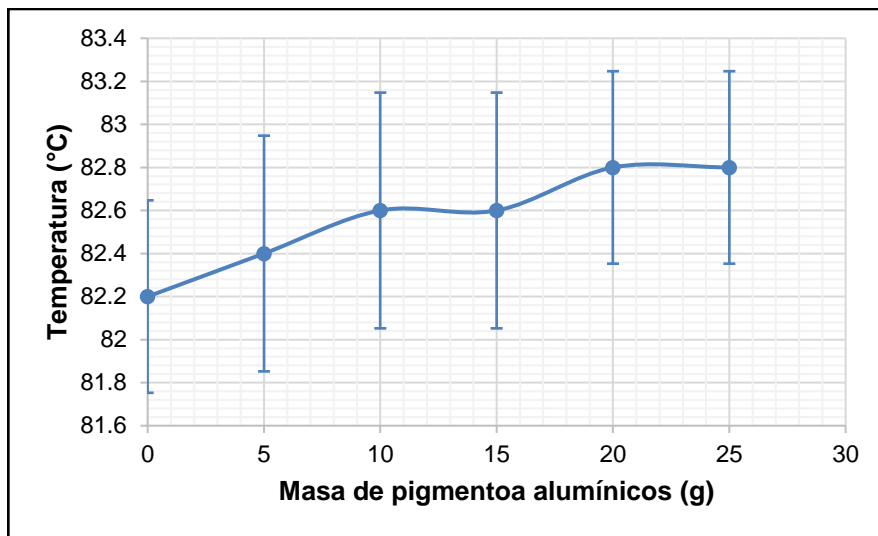
Figura 4. Ascenso de la temperatura de ebullición para el solvente isopropanol
