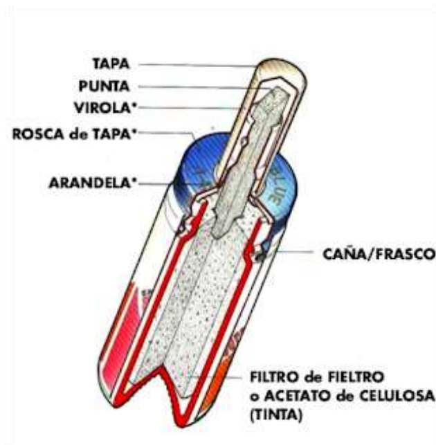
Figura 2. Partes principales del rotulador
