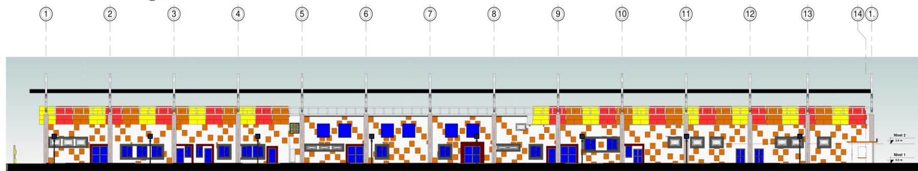
3 01 ELEVACIÓN SUR 1:200
