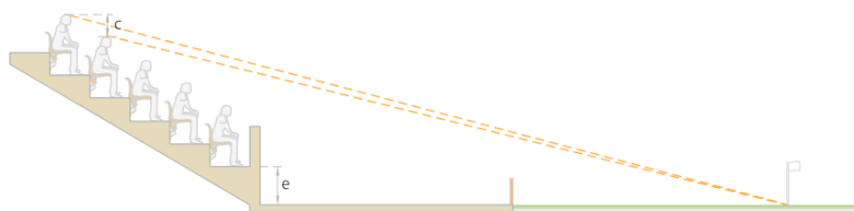
Imagen # 17. Línea de visibilidad. Fuente: Estadios de Fútbol. FIFA, 2019
