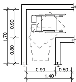
Planta de Pasillos (disposiciones varias)
