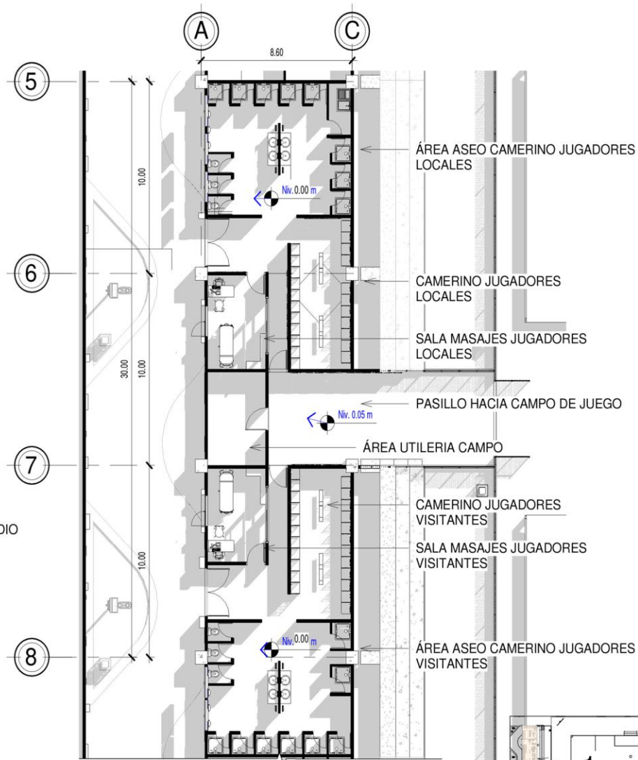
2 02 ÁREA JUGADORES 1 : 200
