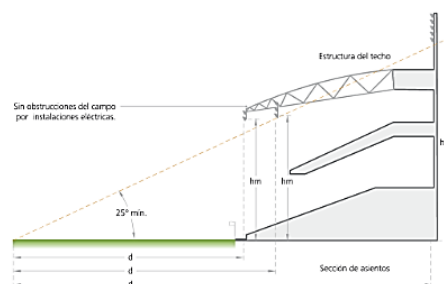
Imagen # 29. Altura de montaje de los aparatos de alumbrado. Fuente: Estadios de Fútbol. FIFA, 2019
