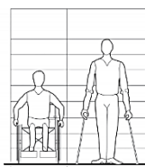
Pasillo p/silla de ruedas y circulación frontal mínima con uso de auxiliar
