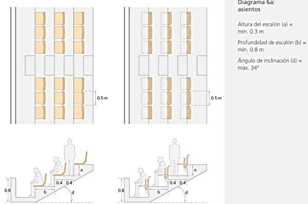
Imagen # 16. Diagrama de asientos. Fuente: Estadios de Fútbol. FIFA, 2019
