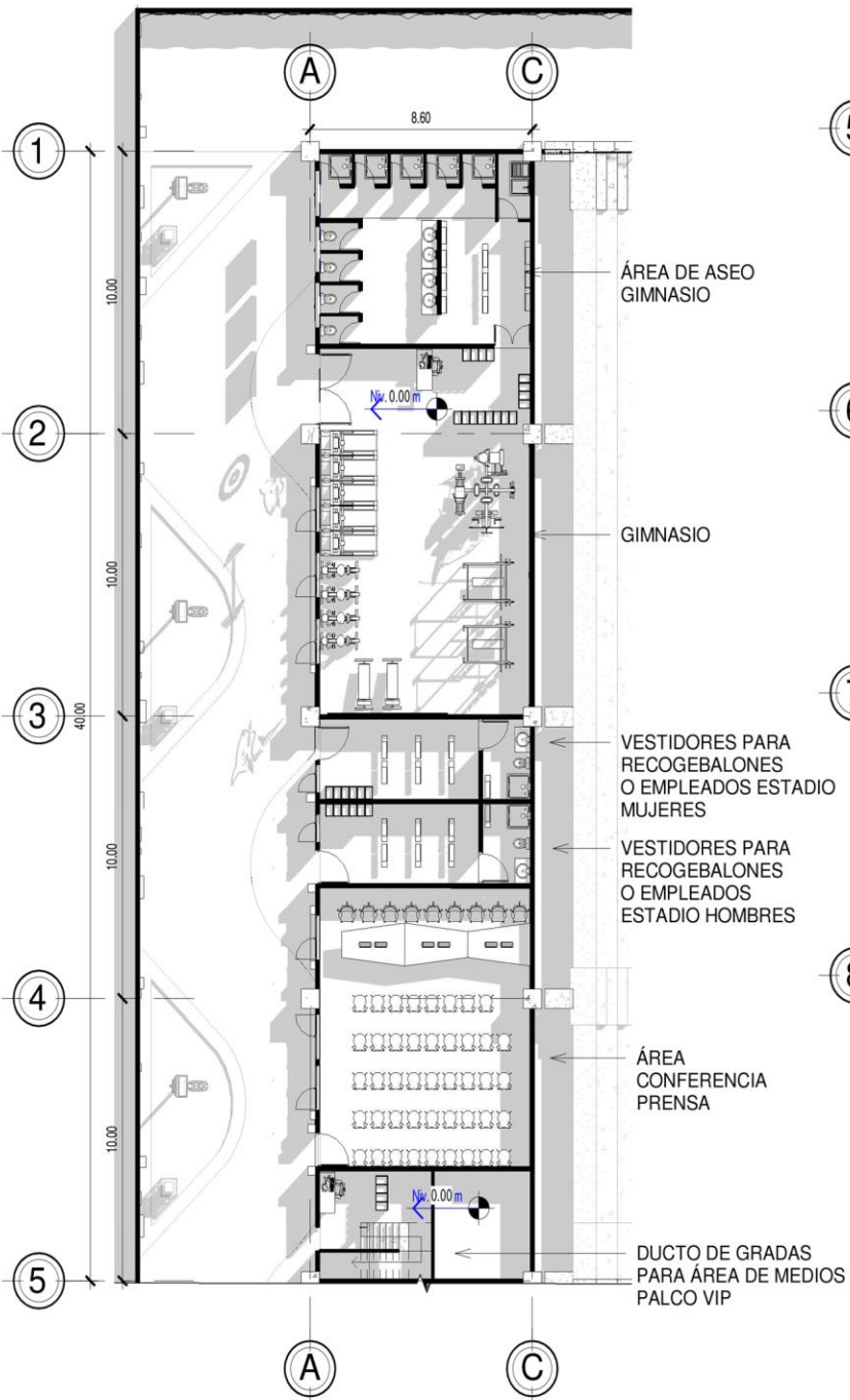
1 01 ÁREA JUGADORES 1 : 200
