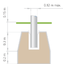
Cimientos del poste
