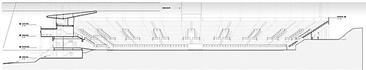
Sección # 3, Sección transversal del complejo deportivo. Fuente: Plataforma Arquitectura, 2019
