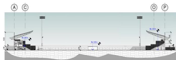
2 01 SECCIÓN GRADERÍOS 1 : 500
