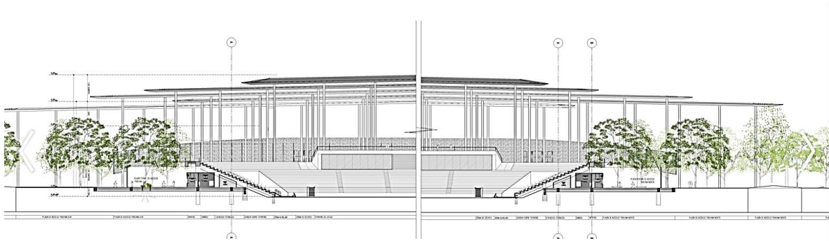
Sección # 2, Sección general del complejo deportivo. Fuente: Plataforma Arquitectura, 2019
