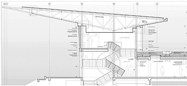
Sección # 4, Sección del bloque donde se ubican los ambientes arquitectónicos. Fuente: Plataforma Arquitectura, 2019
