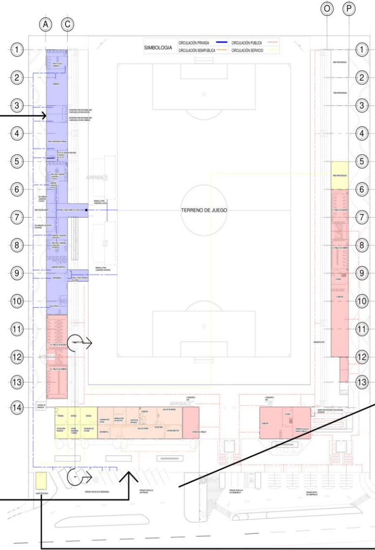
1 PLANTA DE CIRCULACIONES 1 : 500
