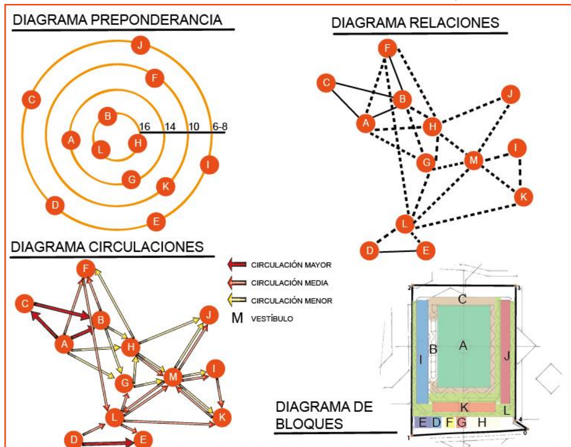
Diagramas # 2. Diagramas de preponderancia, relaciones, circulaciones y bloques de áreas exteriores para el anteproyecto del estadio municipal. Municipio de Sipacate, Escuintla. Fuente: elaboración propia, 2020
