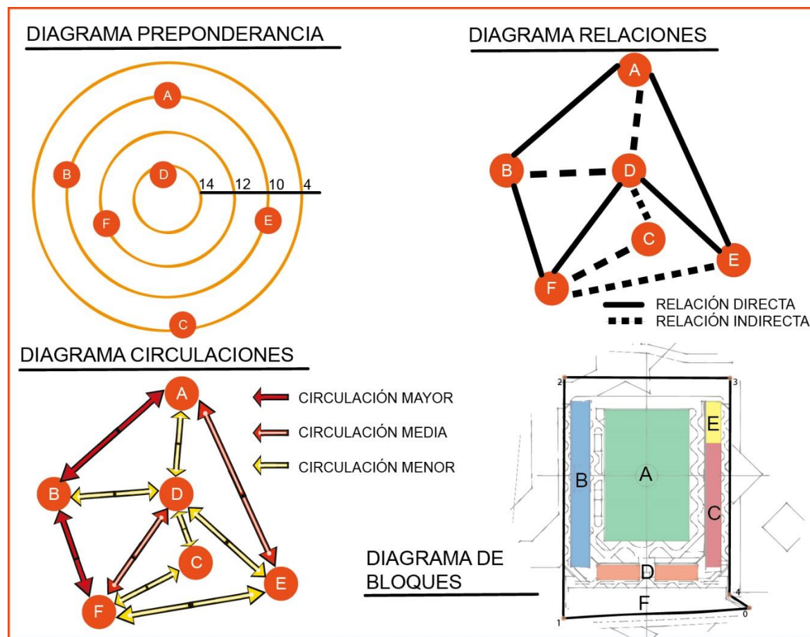
Diagrama # 1. Diagramas de preponderancia, relaciones, circulaciones y bloques de áreas generales para el anteproyecto del estadio municipal. Municipio de Sipacate, Escuintla. Fuente: elaboración propia, 2020
