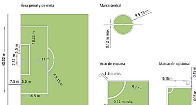
Imagen # 4. Detalles del terreno de juego. Fuente: Estadios de Fútbol. FIFA, 2019
