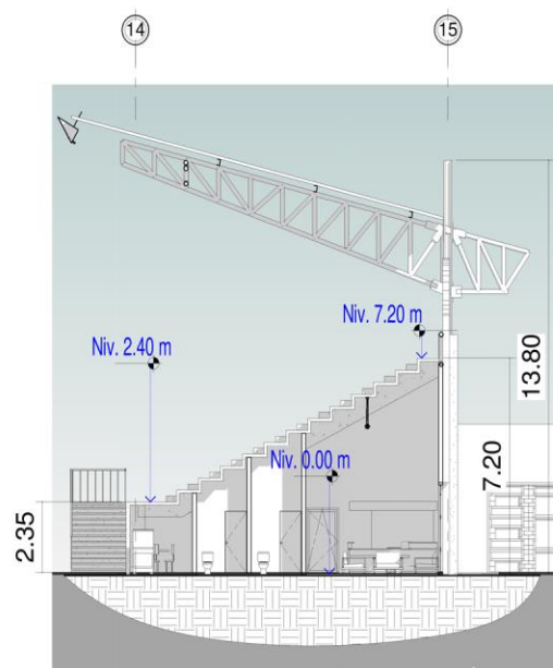
4 03 SECCIÓN GRADERIO SUR 1 : 100
