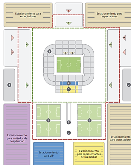
Imagen # 2. Zonas de un estadio. Fuente: Estadios de Fútbol. FIFA, 2019
