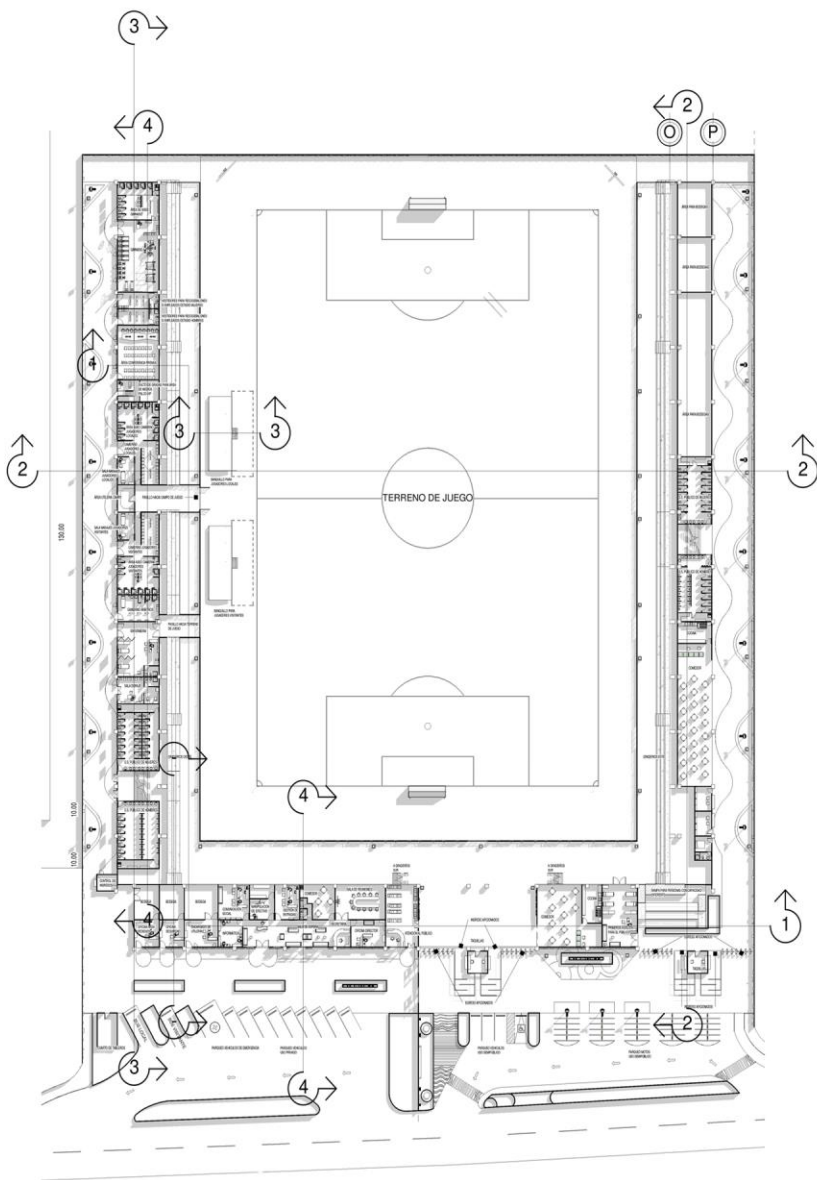
1 PLANTA DE CONJUNTO 1 : 500
