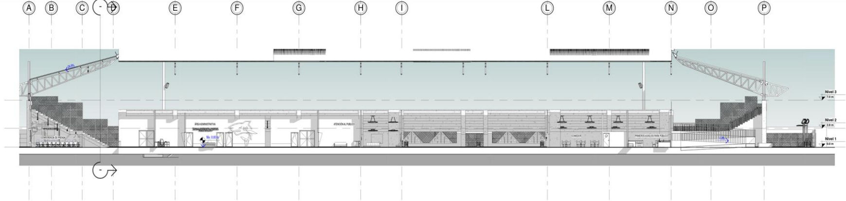
1 01 SECCIÓN GRADERIO OESTE Y ÁREA ADMINISTRATIVA
