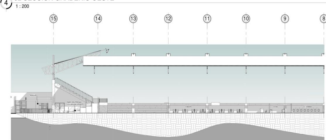
4 02 SECCIÓN GRADERIO OESTE
