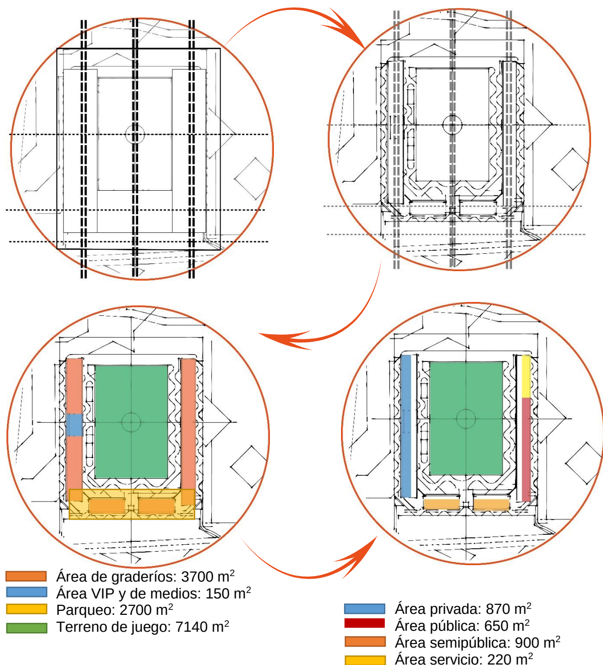
Esquema # 9. Bloques de forma para el anteproyecto del estadio municipal. Municipio de Sipacate, Escuintla. Fuente: elaboración propia, 2020
