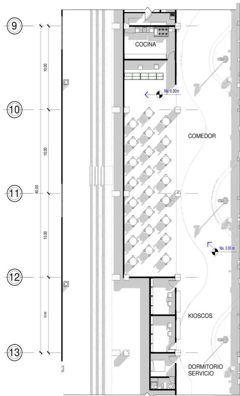
7 07 ÁREA ESPECTADORES 1 : 200
