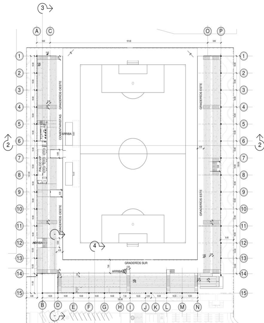
1 PLANTA DE GRADERÍOS 1 : 500
