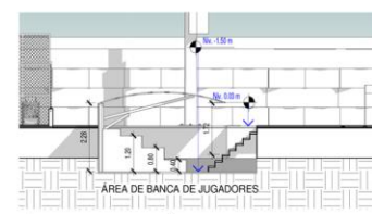
3 04 SECCIÓN BANCA DE JUGADORES
