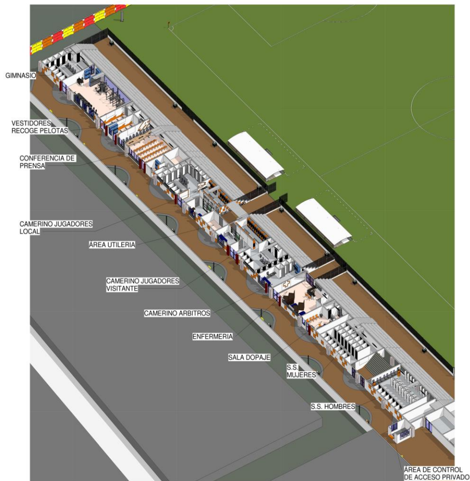
2 01 PLANTA 3D
