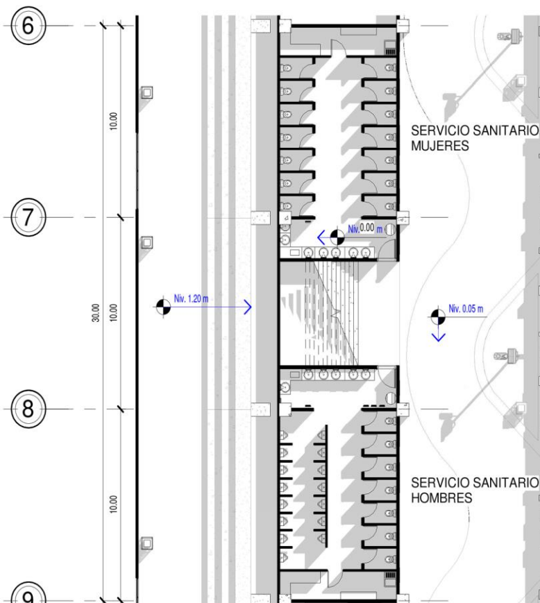
8 06 ÁREA ESPECTADORES 1 : 200
