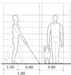
Pasillo con área mínima p/circulación con perro guía
