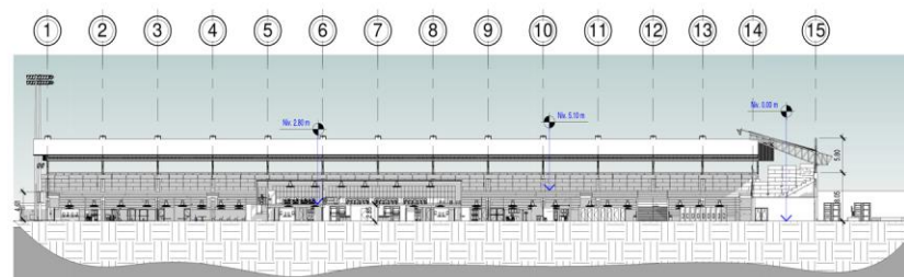
3 02 SECCIÓN GRADERÍOS OESTE 1 : 500
