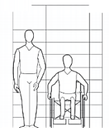
Pasillo p/silla de ruedas y circulación frontal mínima
