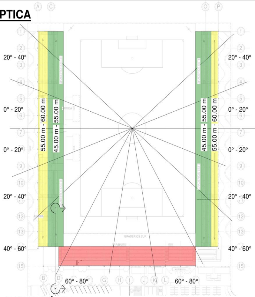
1 PLANTA DE ISÓPTICA 1 : 500
