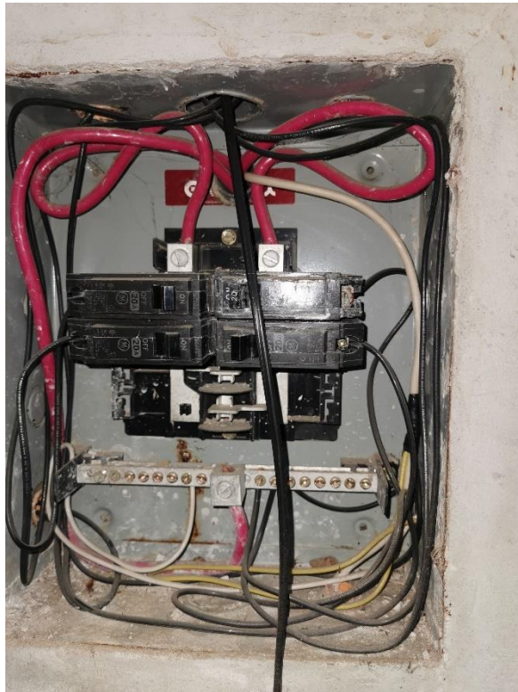
Figura 23. Tablero de distribución secundario Museo del Libro Antiguo
