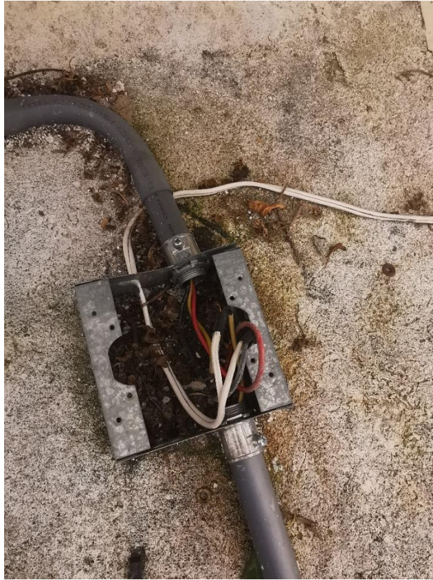
Figura 25. Caja de registro con instalación defectuosa
