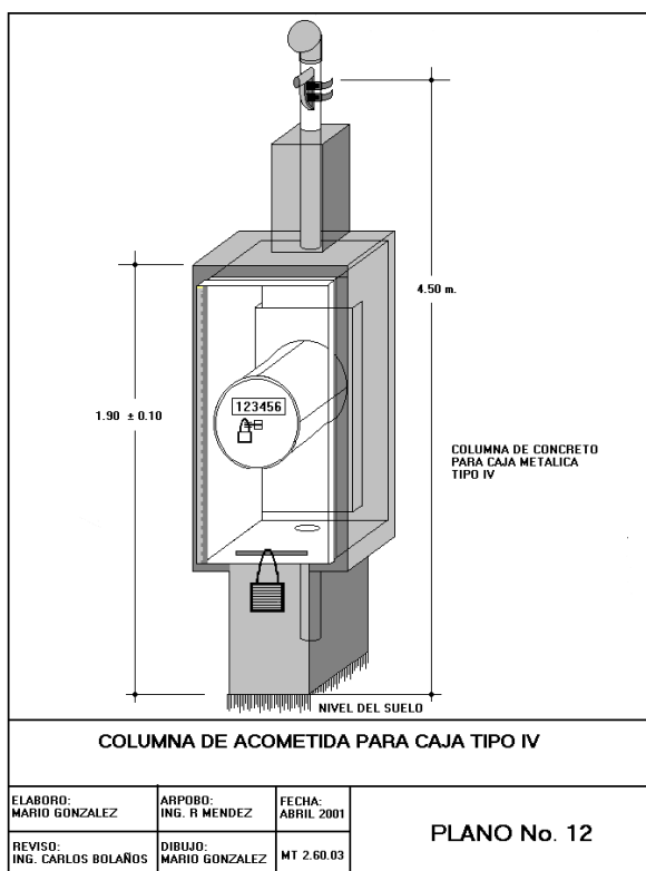
Figura 5. Esquema de acometida según EEGSA cargas monofásicas entre 10 y 25 KVA
