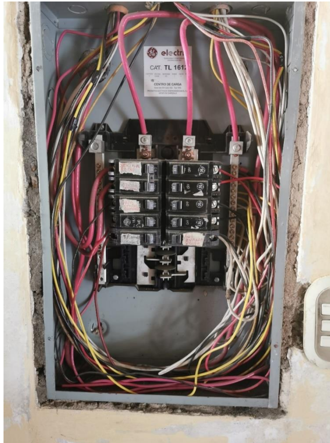
Figura 22. Tablero principal de distribución Museo del Libro Antiguo
