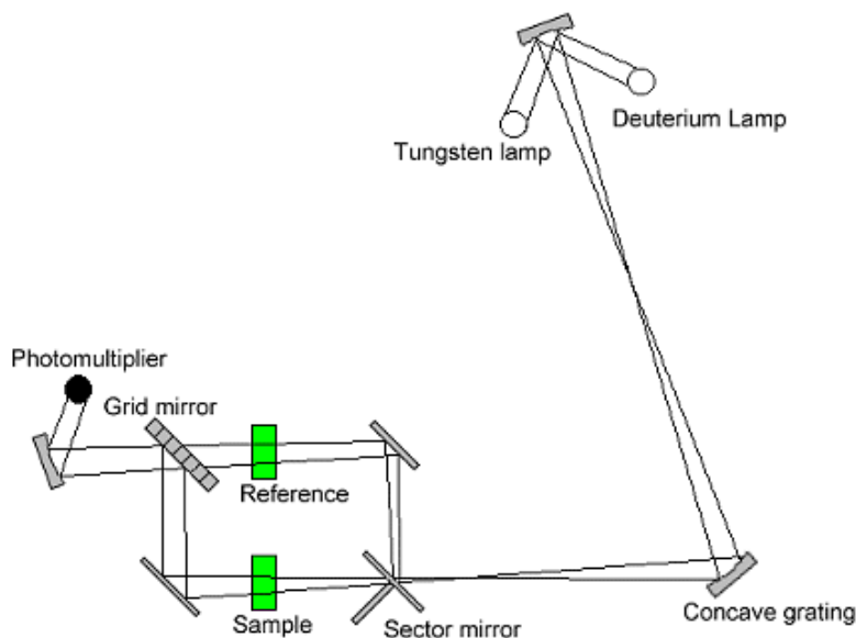
Figura 16. Esquema gráfico de funcionamiento interno espectrofotómetro UV-VIS doble haz
