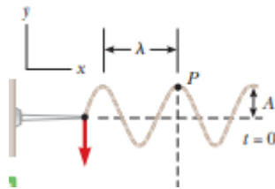
Figura 2. Características de una onda
