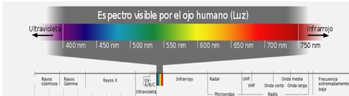
Figura 4. Espectro electromagnético
