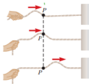
Figura 1. Ondas en una cuerda
