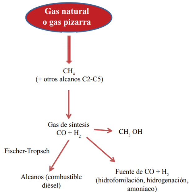
Figura 1. Proceso Fischer-Tropsch
