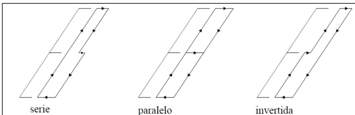
Figura 13. Configuraciones de ciclos de absorción de doble efecto
