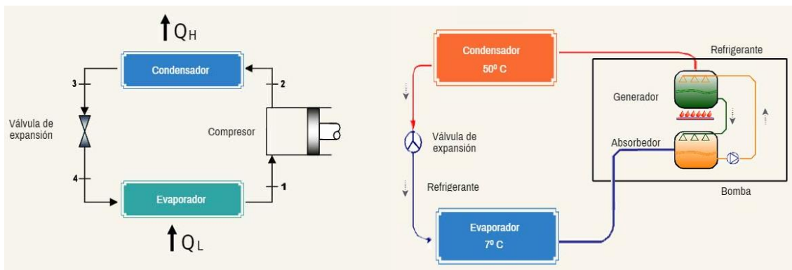
Figura 14. Comparación de un sistema por compresión frente a un sistema por absorción
