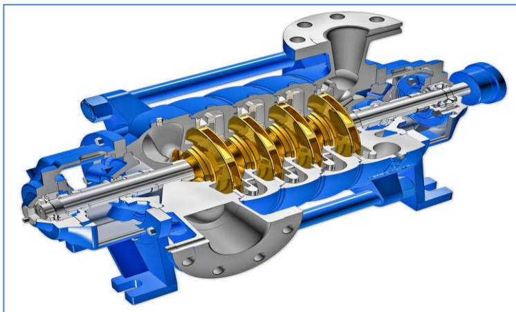
Figura 2. Bomba de 4 etapas
