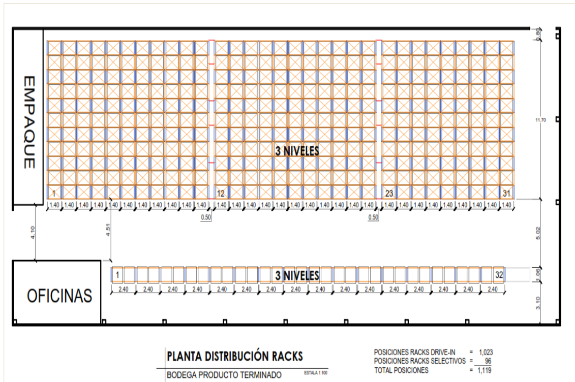
Figura 13. Plano distribución de racks
