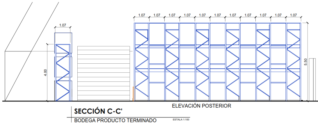
Figura 18. Detalle racks elevación posterior
