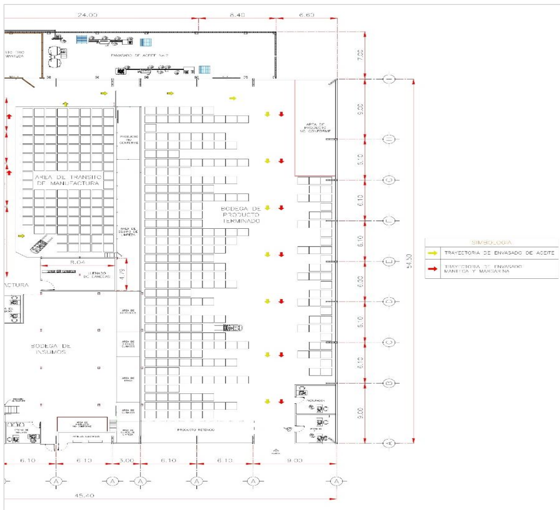
Figura 12. Diagrama de recorrido
