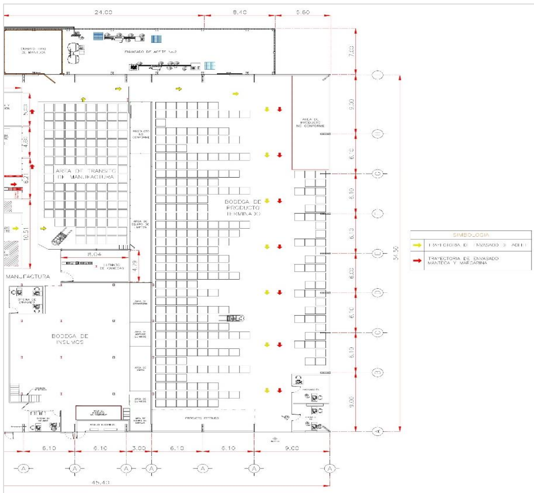
Figura 20. Diagrama de recorrido
