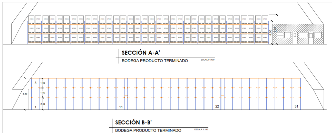
Figura 14. Racks sección A y sección B
