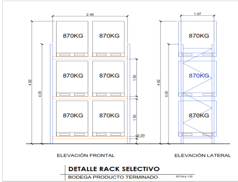
Figura 16. Detalle racks selectivo
