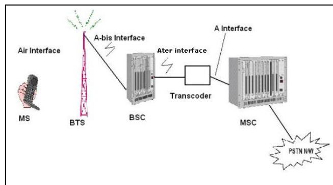
Figura 38. Interfaces A-ter
