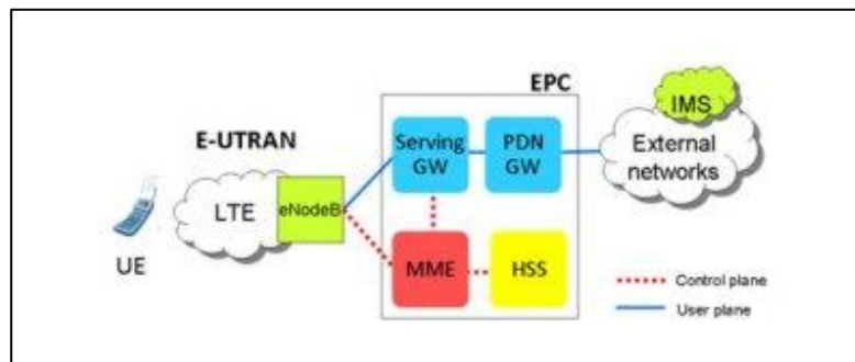
Figura 59. Arquitectura EPS básica con E-UTRAN Access
