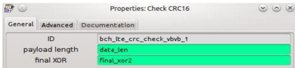
Figura 122. Configuración bloque Check CRC16
