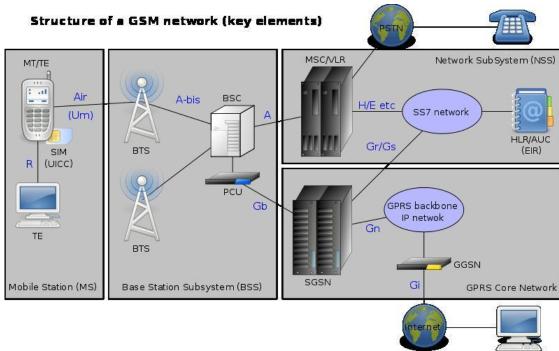
Figura 33. Esquema general de una red GSM
