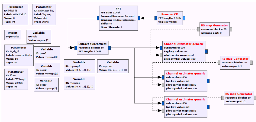
Figura 98. Diagrama de bloques recepción OFDM
