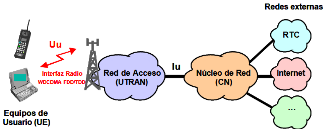
Figura 48. Arquitectura genérica UMTS
