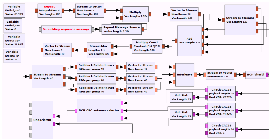
Figura 109. Diagrama de flujo de decodificación BCH y MIB
