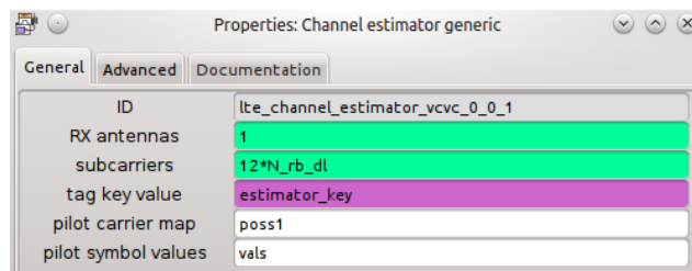
Figura 100. Configuración de bloque Channel estimator generic
