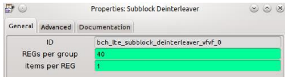
Figura 120. Configuración bloque Subblock deinterleaver
