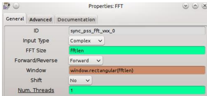
Figura 88. Configuración FFT
