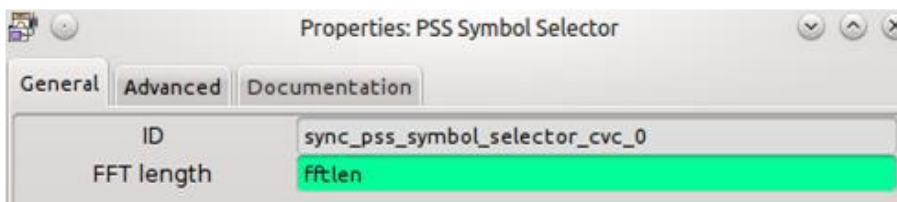
Figura 87. Configuración bloque PSS Symbol Selector
