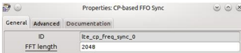
Figura 86. Configuración bloque CP-based FFO Sync
