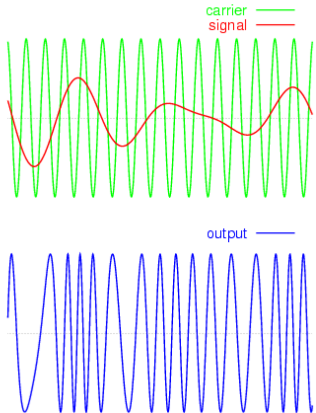
Figura 12. Modulación de frecuencia
