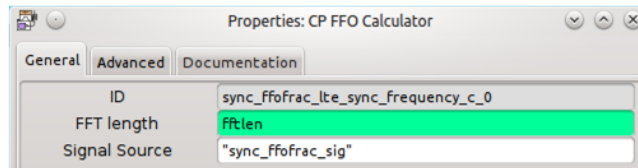
Figura 94. Configuración de bloques CP FFO Calculator
