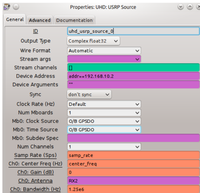
Figura 82. Configuración bloque UHD-USRP Source
