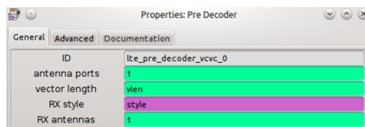
Figura 105. Configuración de bloque Pre Decoder
