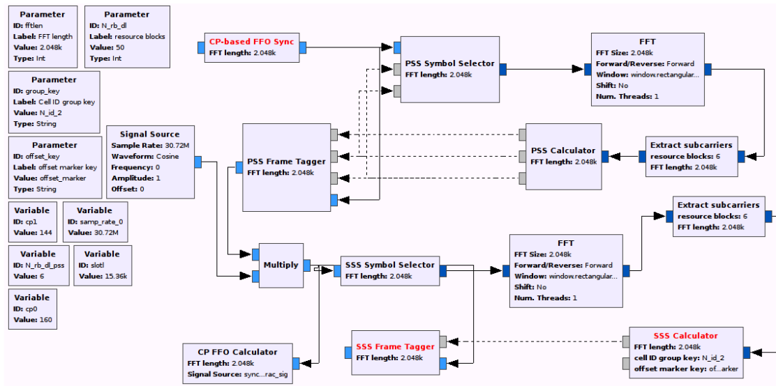
Figura 85. Diagrama de bloques de sincronización
