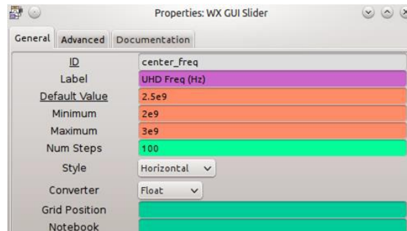
Figura 83. Configuración de bloque WX GUI Slider
