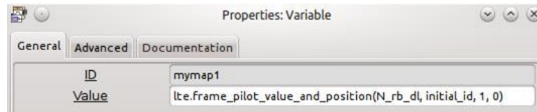
Figura 102. Configuración de variable importación LTE
