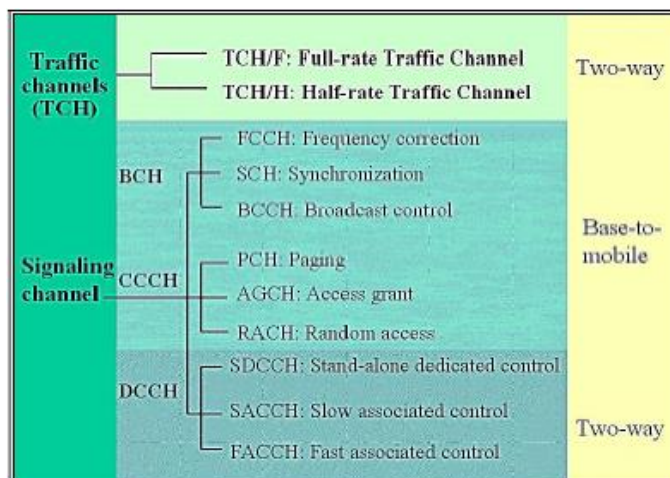
Figura 18. Radio canales
