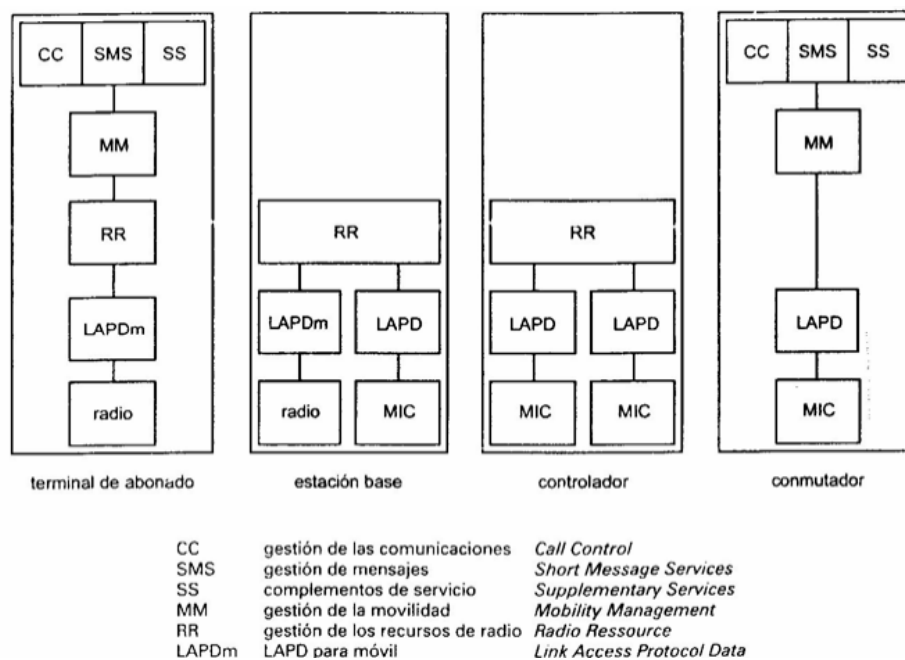
Figura 34. Protocolos en una estación móvil y el subsistema de radio
