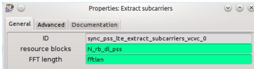
Figura 89. Configuración de bloque Extract subcarriers
