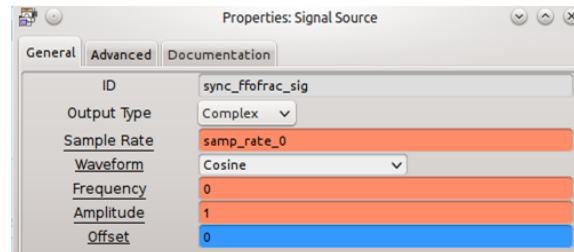
Figura 92. Configuración de bloque Signal Source
