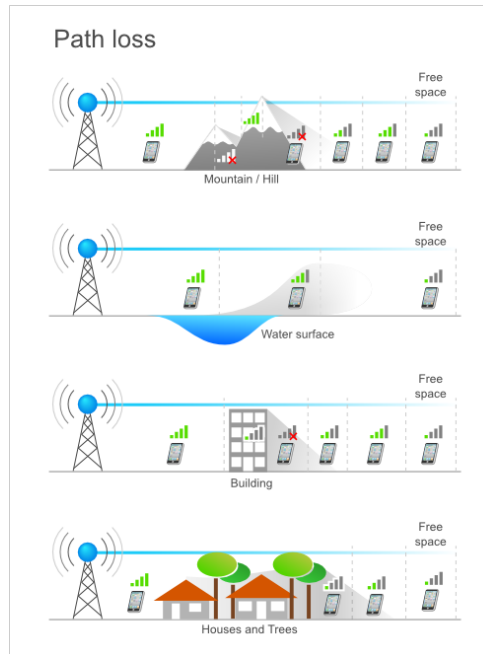
Figura 61. Pérdida de trayectoria ( Path Loss )
