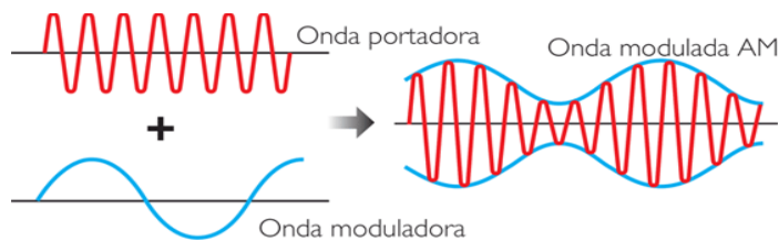
Figura 11. Modulación en amplitud
