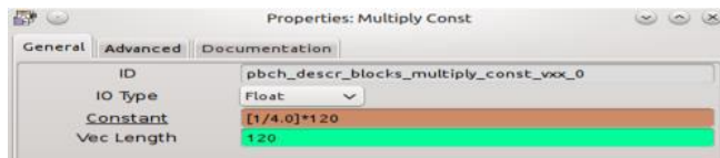
Figura 118. Configuración bloque Multiply Const
