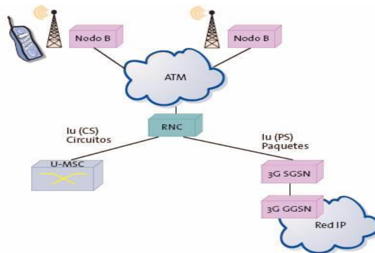
Figura 46. Estructura UMTS
