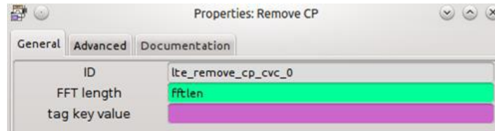
Figura 99. Configuración de bloque Remove CP
