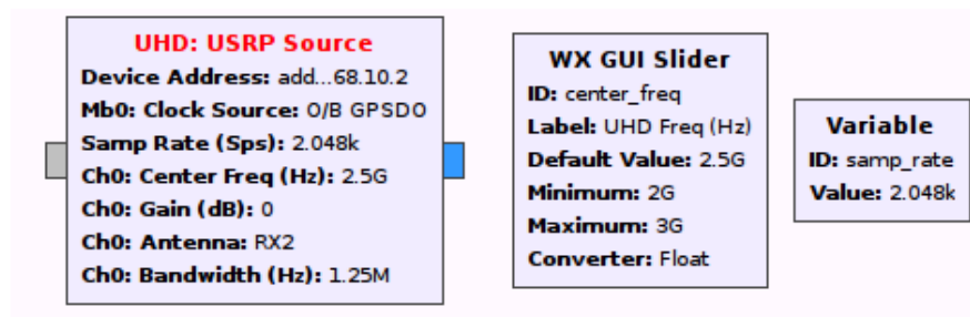
Figura 81. Bloque de conexión USRP N210 con GNURadio
