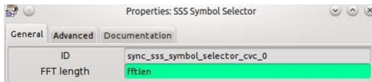
Figura 95. Configuración de bloque SSS Symbol Selector
