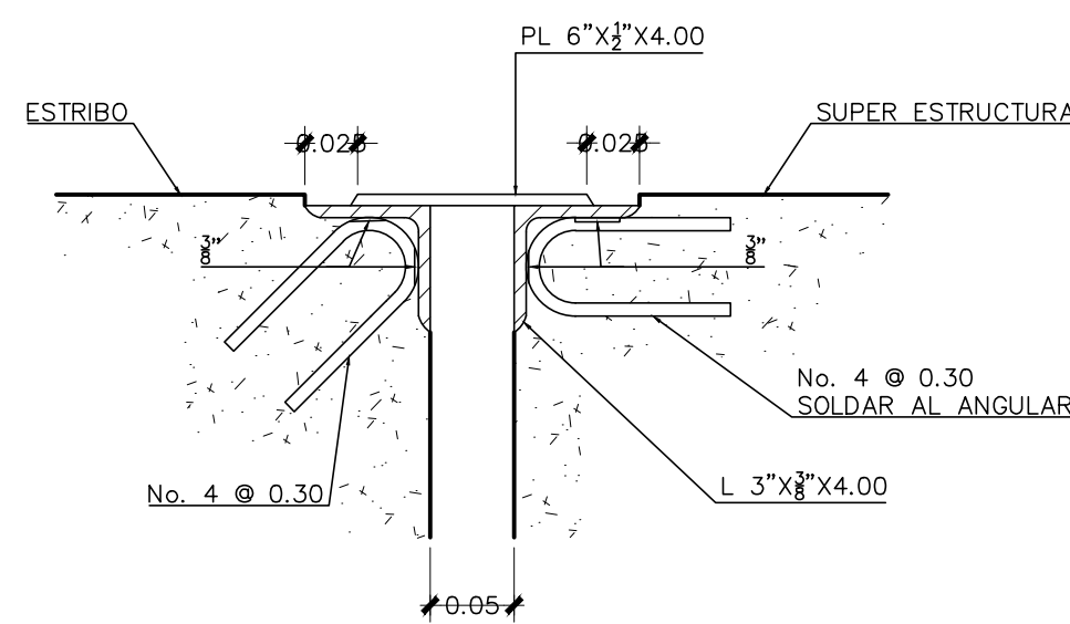
DETALLE DE JUNTA DE CALZADA
