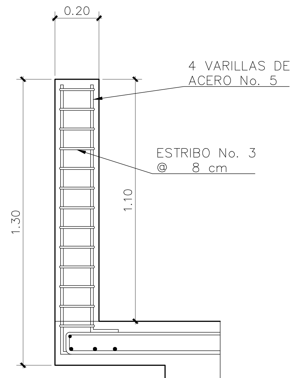
DETALLE DE BARANDAL
