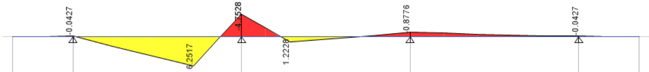
Figura 10. Diagrama de momento por camión HL-93
