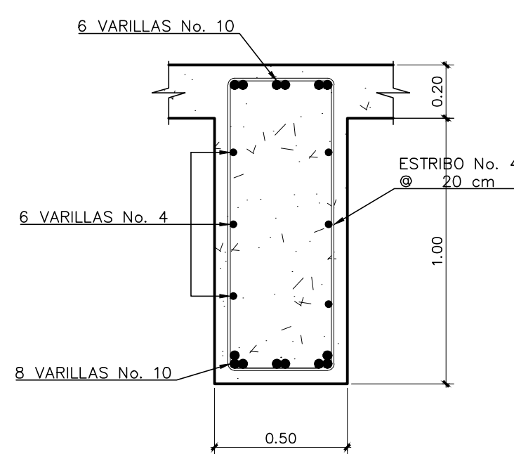
VIGA INTERIOR
