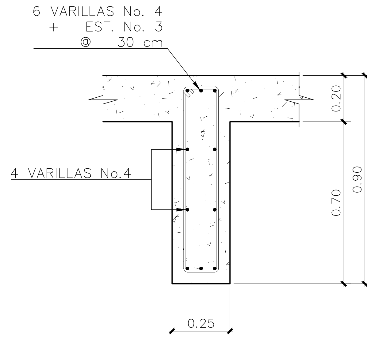
DIAFRAGMA INTERNO
