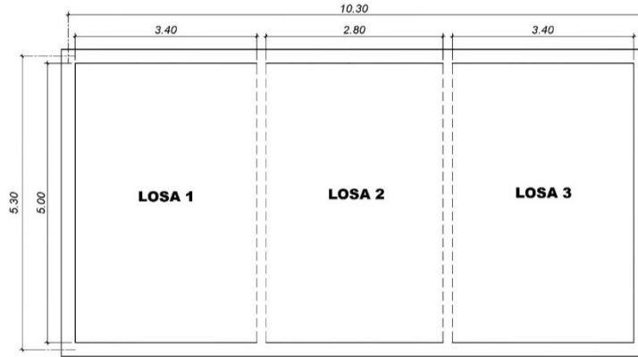
Figura 3. Distribución de losas del tanque de distribución
