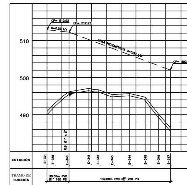
PERFIL LD – RAMAL 14.2
