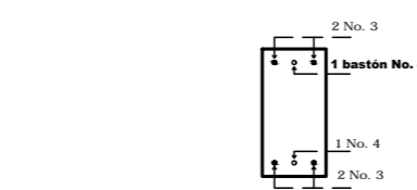
SECCIÓN C - C' DE VIGA
