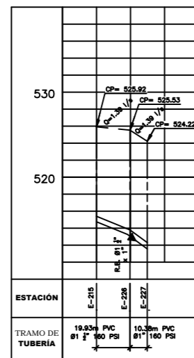
PERFIL LD – RAMAL 8.2
