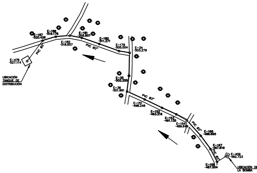
PLANTA LÍNEA DE IMPULSIÓN
