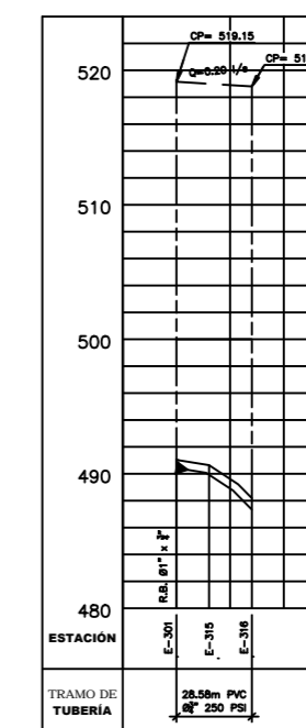
PERFIL LD – RAMAL 13.1
