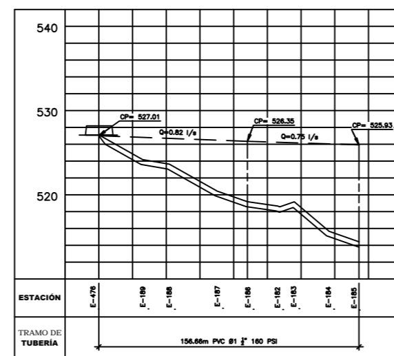
PERFIL LD – RAMAL 7
