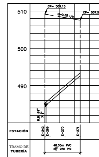
PERFIL LD – RAMAL 9.2
