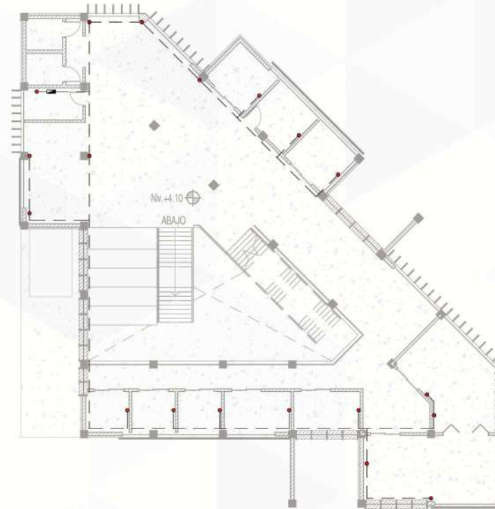
PISO 02 - ESQUEMA FUERZA 1 : 300
