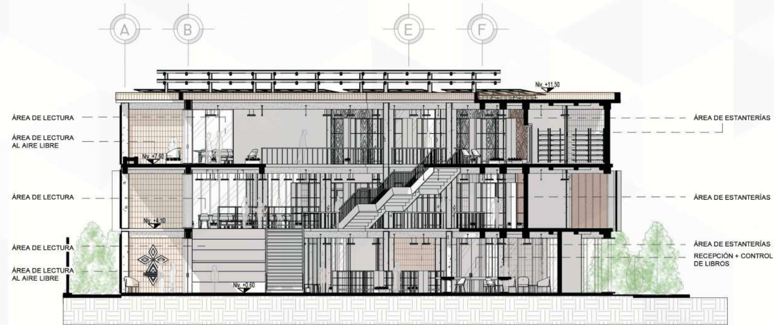
SECCIÓN A 1 : 200
