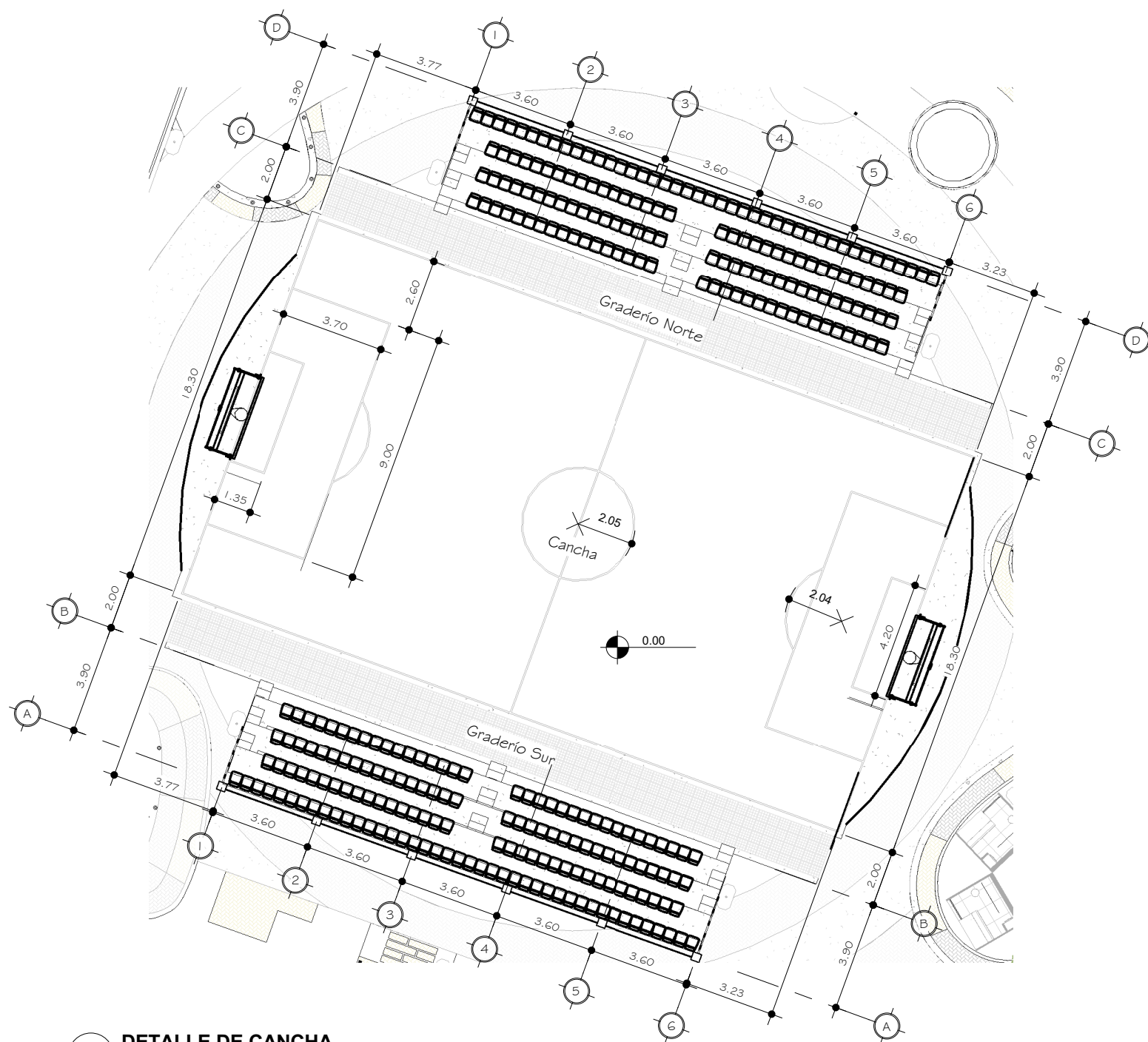
1 DETALLE DE CANCHA
