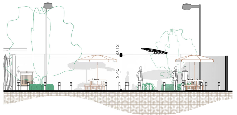
3 ELEVACIÓN - ÁREA DE MESAS INGRESO DETALLE EN SECCION ESC 1 : 150
