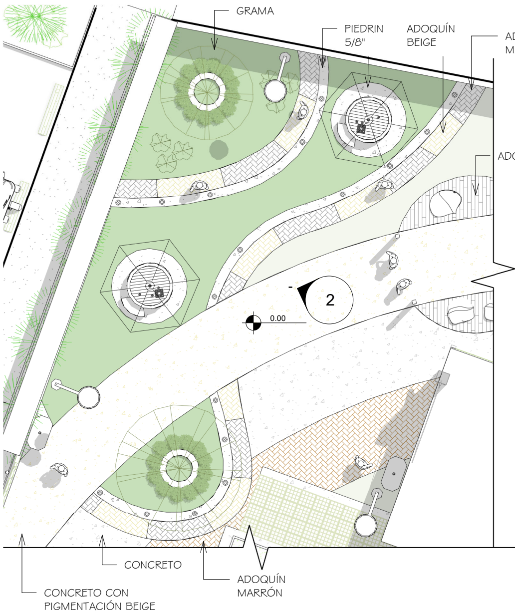
1 ÁREA DE MESAS INGRESO DETALLE EN PLANTA ESC 1 : 100
