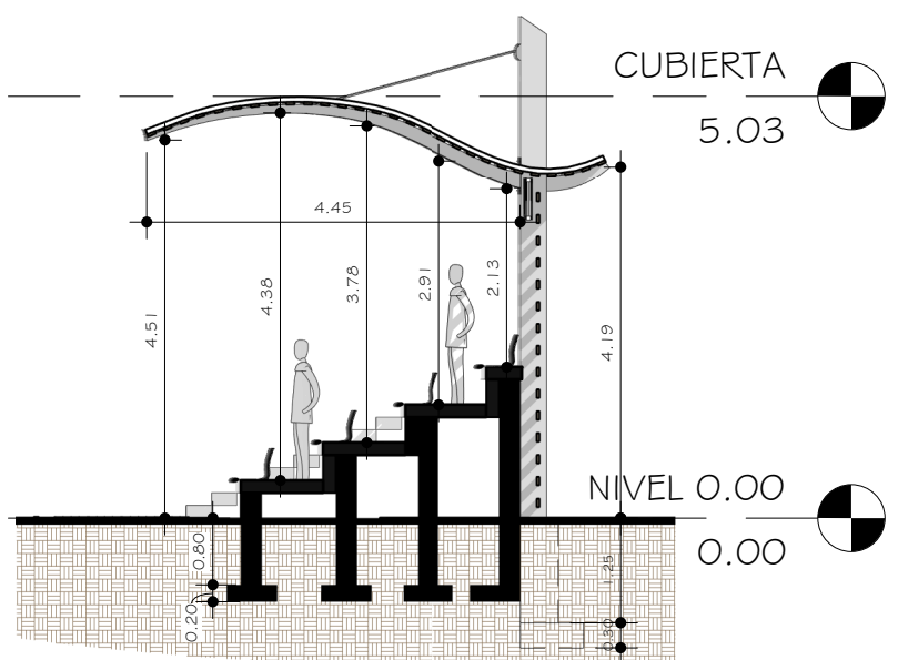
3 SECCIÓN LATERAL - GRADERÍO
