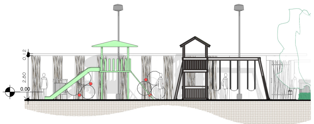
4 ELEVACIÓN - ÁREA DE JUEGOS DETALLE EN SECCION ESC 1 : 150
