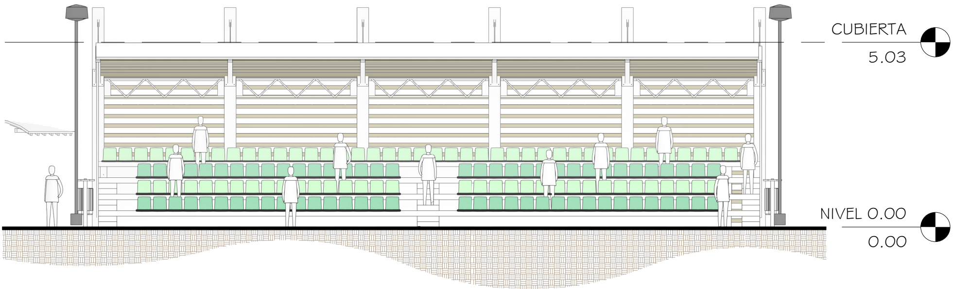
1 ELEVACIÓN FRONTAL - GRADERÍO
