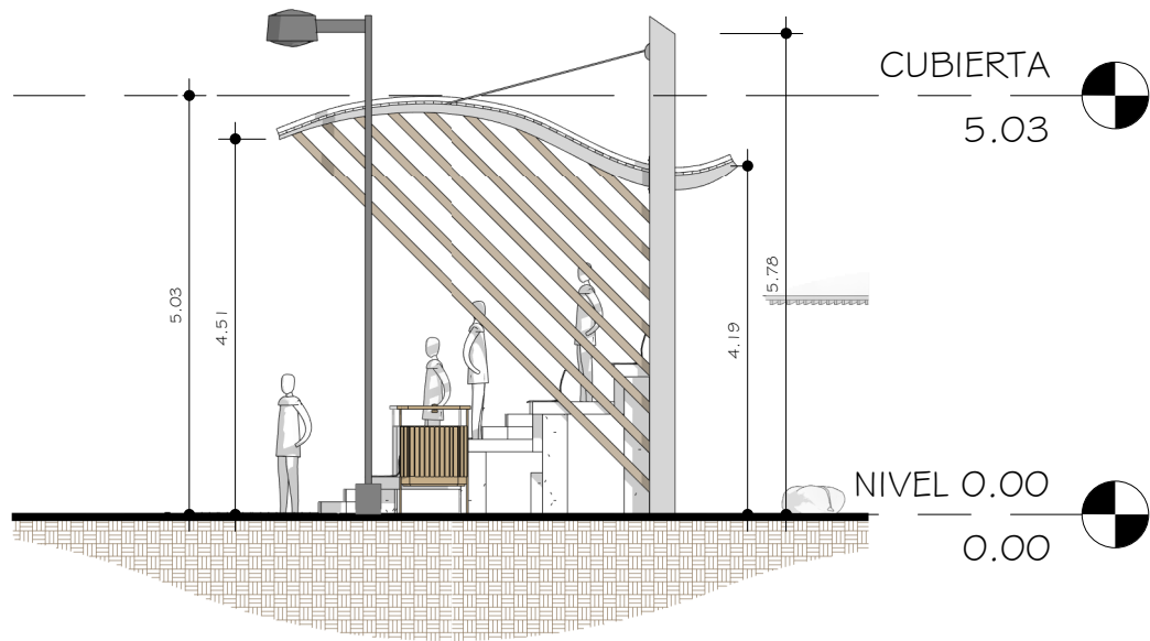
2 ELEVACIÓN LATERAL - GRADERÍO
