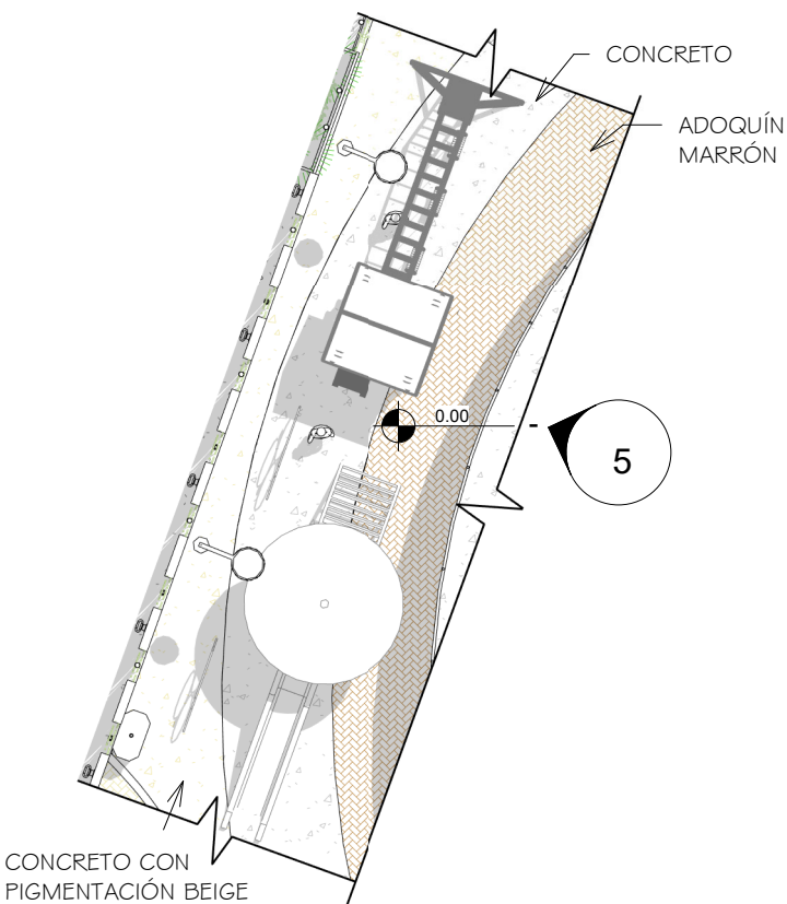
2 ÁREA DE JUEGOS DETALLE EN PLANTA ESC 1 : 150
