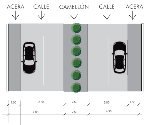
SECCIÓN B'-B'
