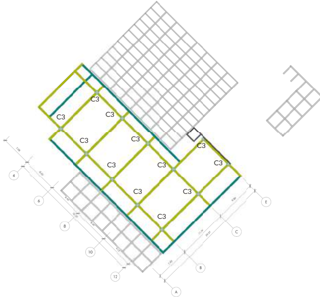
SEGUNDO NIVEL ESQUEMA DE COLUMNAS Y VIGAS
