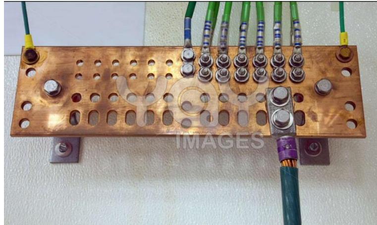
Figura 25. Barra de puesta a tierra
