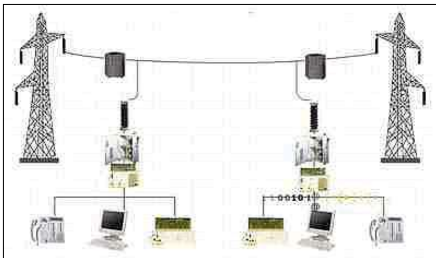
Figura 8. Red PLC comúnmente utilizada en el sistema eléctrico
