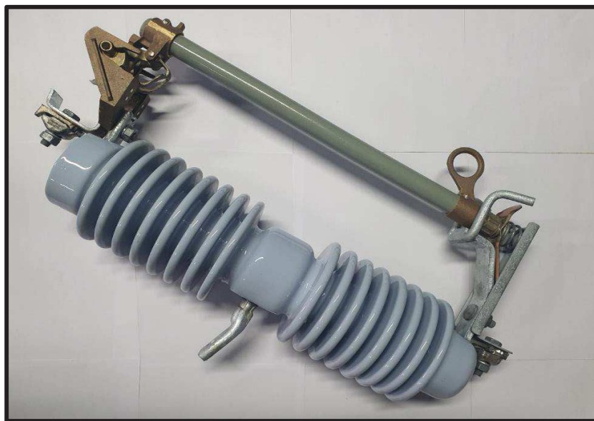
Figura 5. Cortacircuito de porcelana con tubo porta fusible
