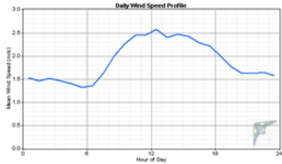
Velocidad del viento 2012, Día
