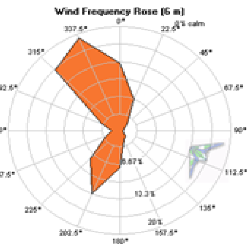
Rosa de vientos año 2012
