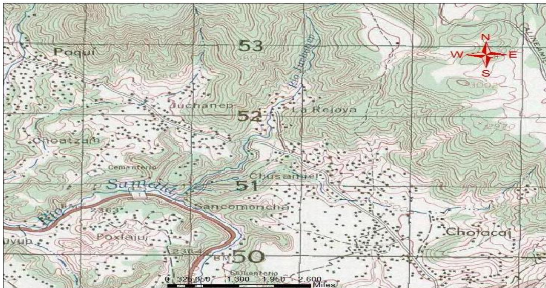
Figura 3: Mapa de curvas de nivel del cantón Juchanep
