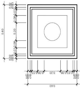
PLANTA DE COLUMNA TIPO-2 ESCALA 1/25
