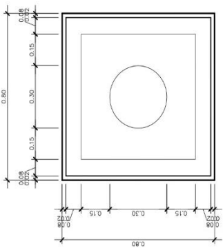
PLANTA DE COLUMNA TIPO-1 ESCALA 1/25
