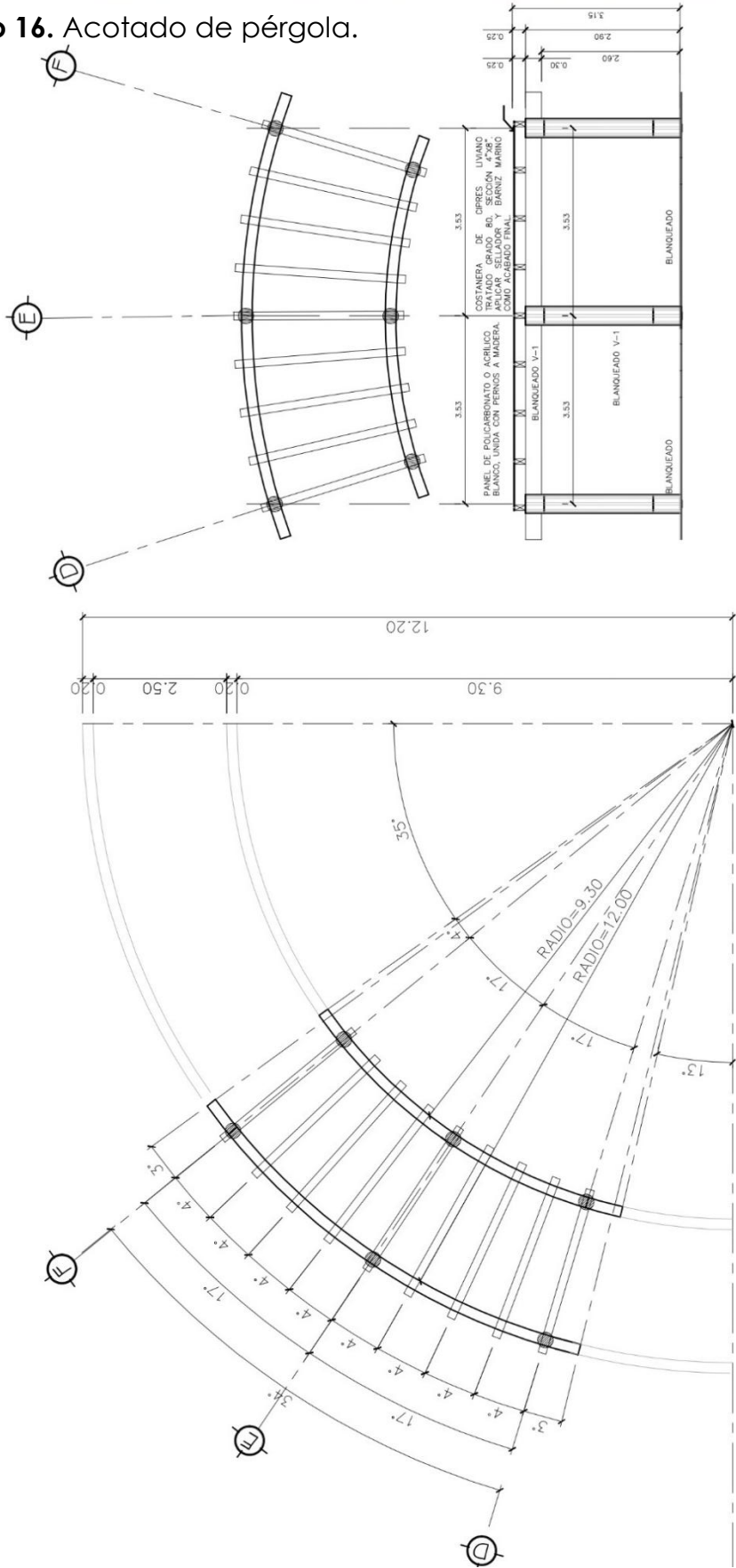
ACOTADO DE PÉRGOLA
