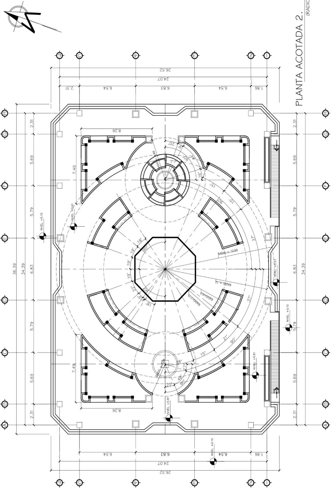
Plano 14. Planta acotada no. 2.
