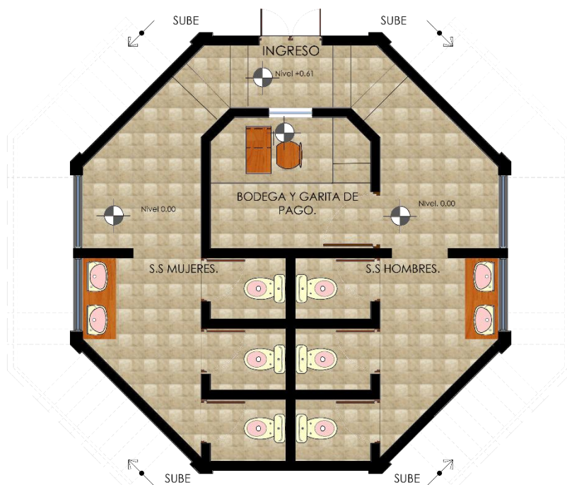
Imagen 19. Kiosco 1er nivel, servicios sanitarios.
