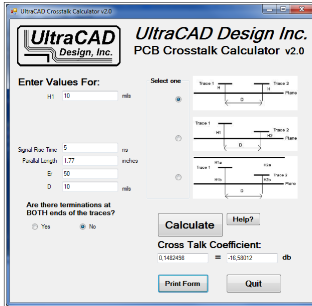
Figura 46. Software ULTRACAD utilizado para medir el crosstalk
