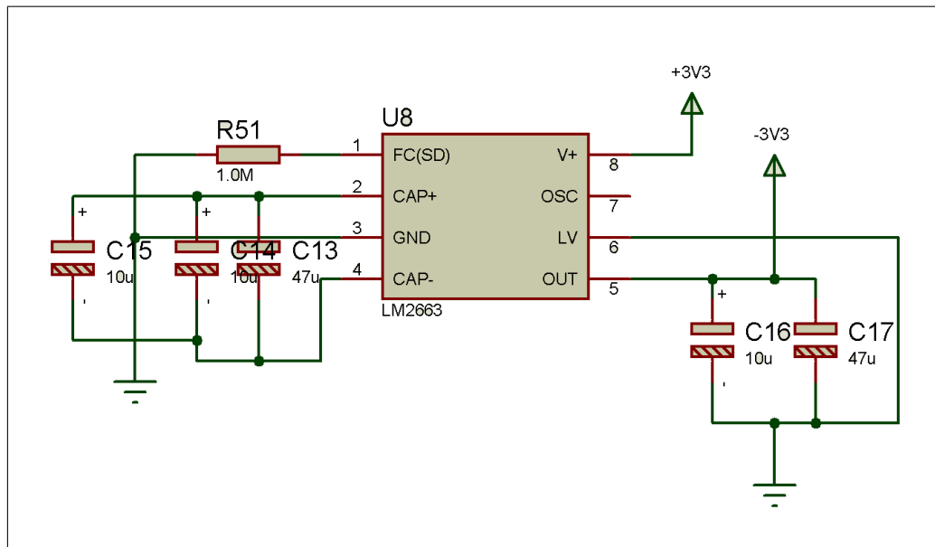
Figura 19. Configuración del inversor de voltaje LM2663
