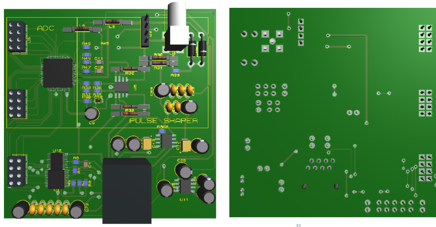
Figura 22. Diseño del prototipo 1 en PCB
