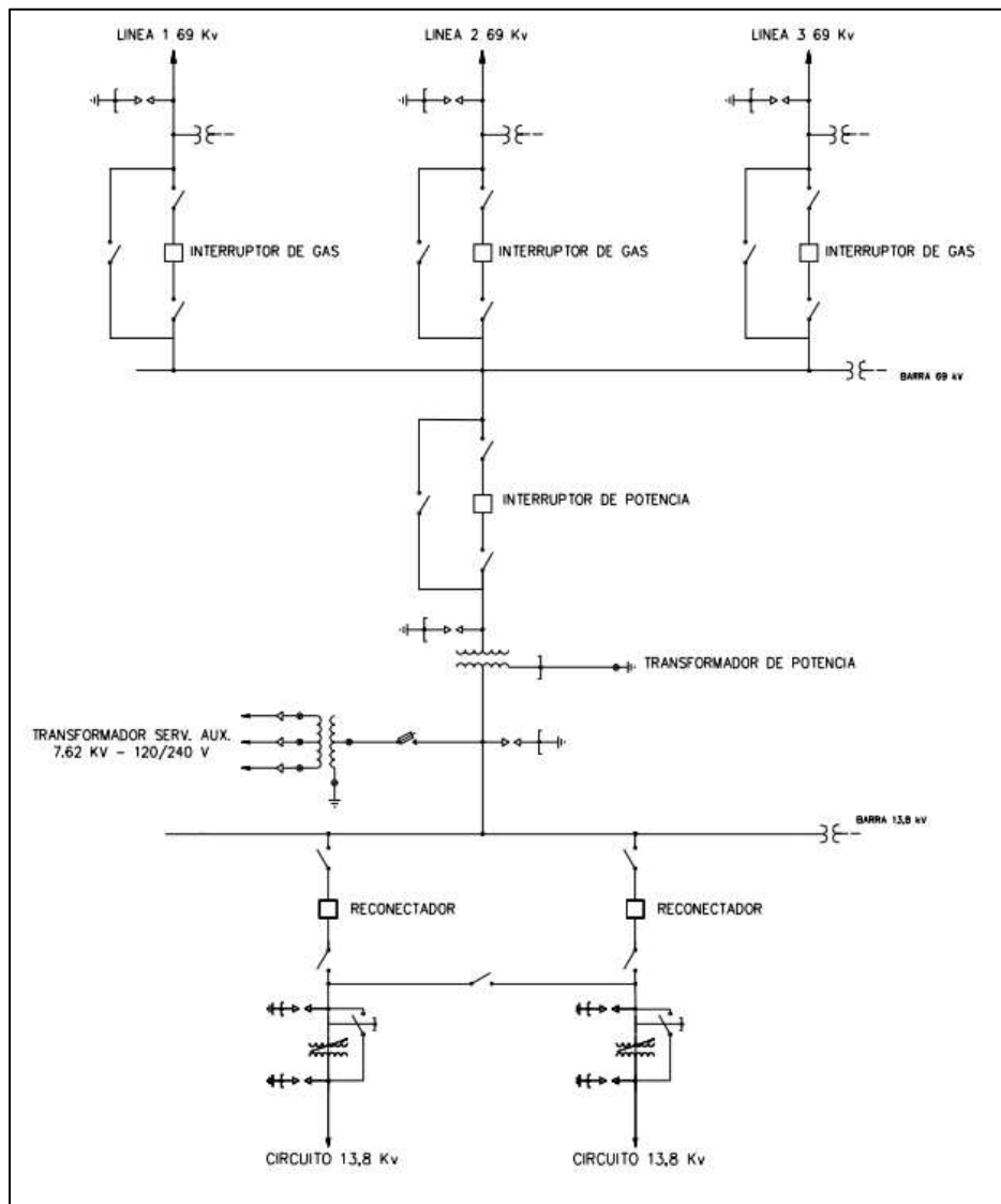
Figura 6. Diagrama unifilar subestación El Milagro
