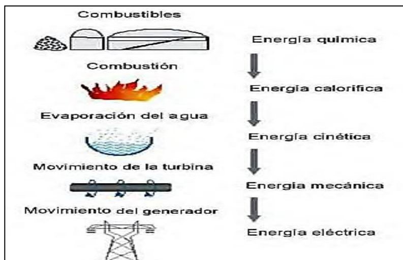
Figura 6. Proceso de la generación de energía en un ingenio azucarero
