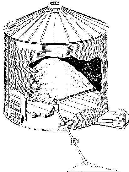
Figura 3. Silo con aireación para almacenamiento de maíz
