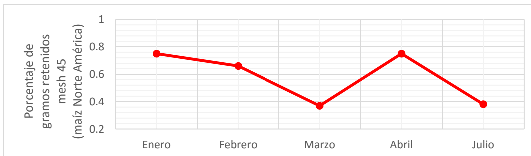
Figura 24. Porcentaje de gramos retenidos en mesh 45 de harina precocida obtenida con maíz proveniente de Norte América
