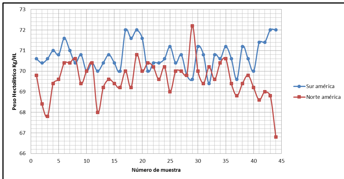
Figura 29. Comparación de peso hectolítrico del maíz de Sur América y Norte América
