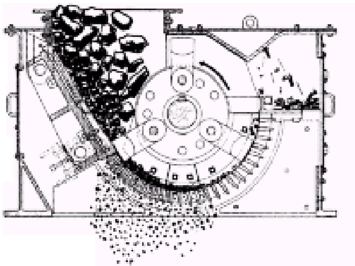
Figura 8. Molino de martillo.
