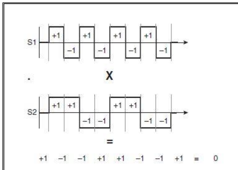
Figura 16. Correlación cruzada de secuencias ortogonales
