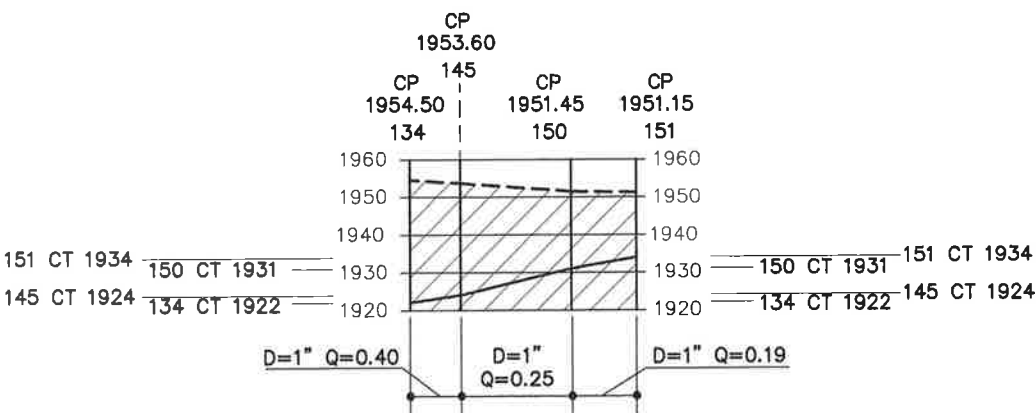
PERFIL F RED DE DISTRIBUCION 1 ESCALA HORIZONTAL 1/4000 ESCALA VERTICAL 1/8000
