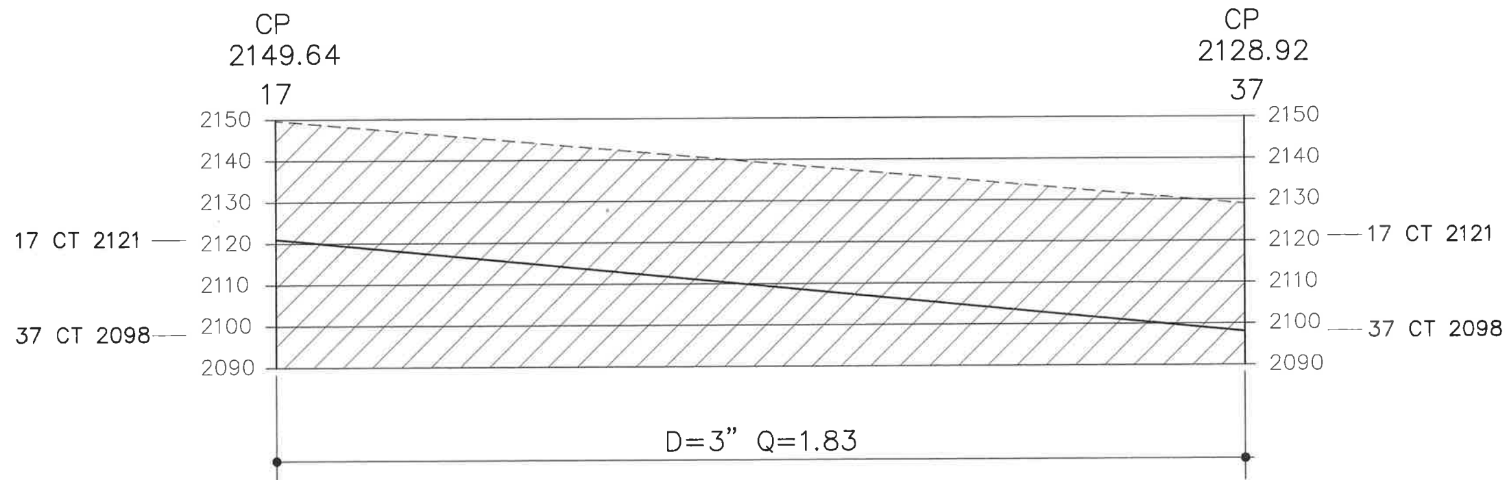
PERFIL LINEA DE CONDUCCION 17 A 37
