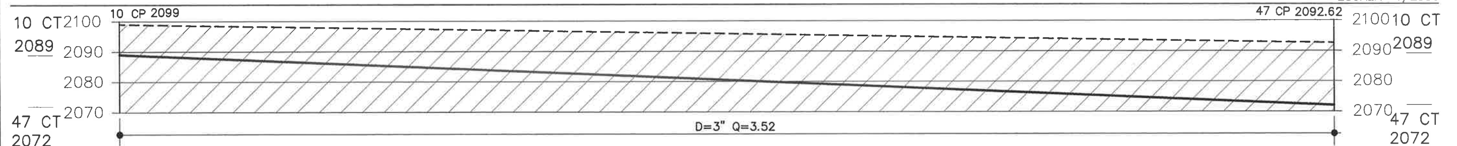
PERFIL LINEA DE CONDUCCION 10 A 47
