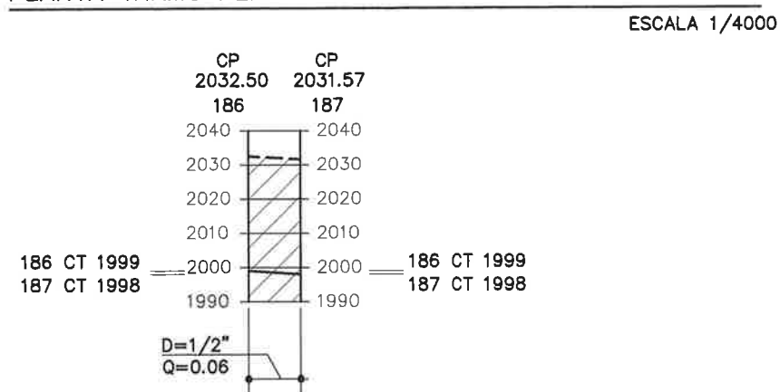
PERFIL "H" RED DE DISTRIBUCION 2 ESCALA HORIZONTAL 1/4000 ESCALA VERTICAL 1/8000
