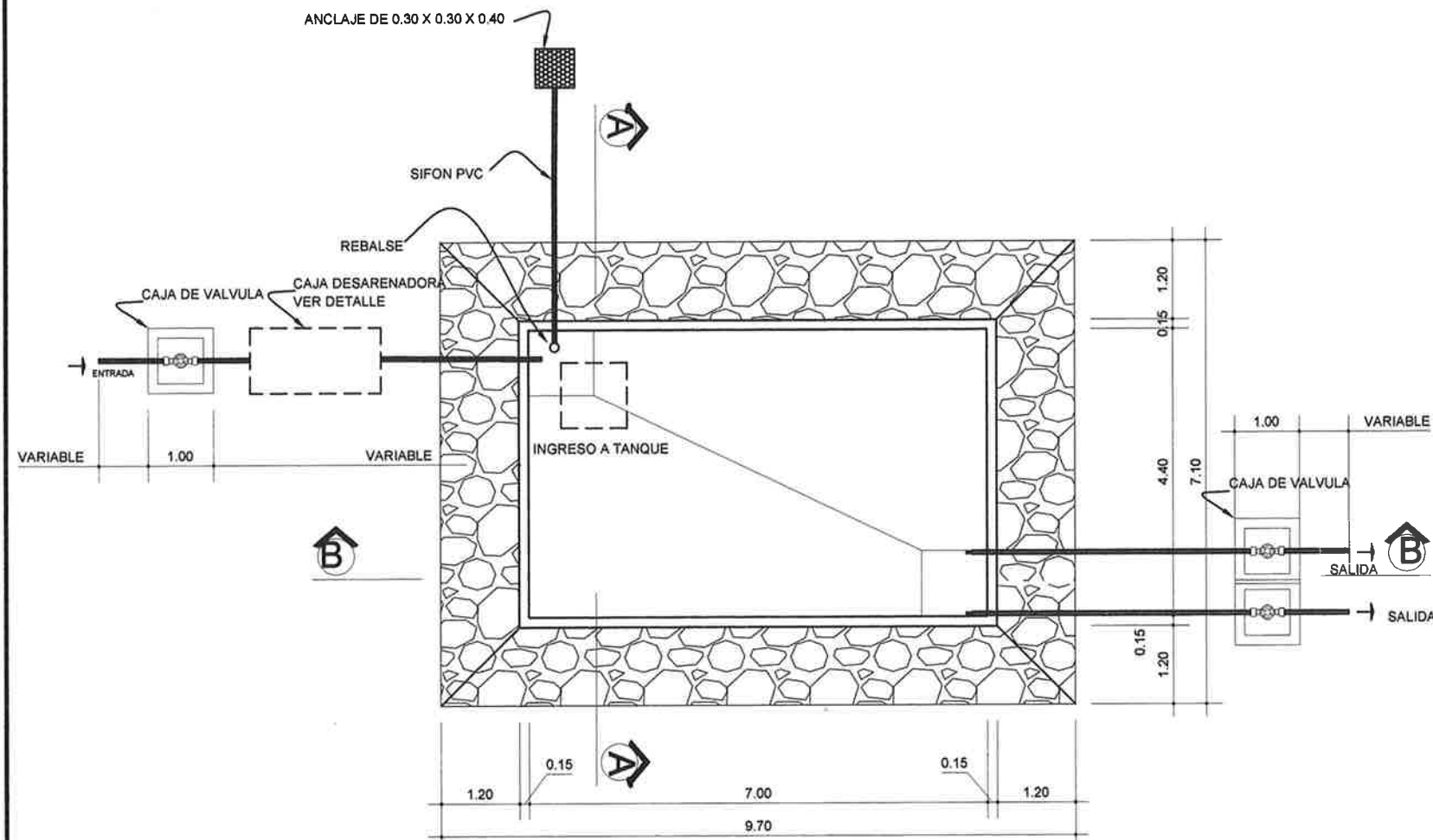
PLANTA GENERAL DE TANQUE DE ALMACENAMIENTO Y DITRIBUCION DE AGUA POTABLE ALDEA SAN MIGUEL
