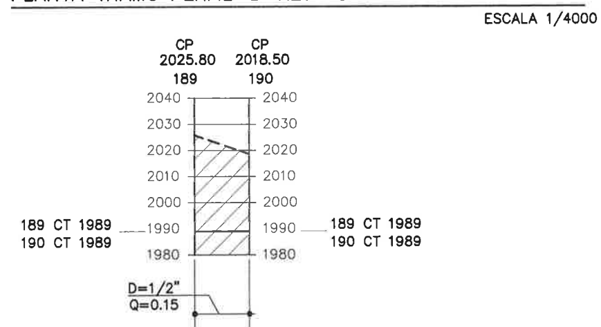
PERFIL "I" RED DE DISTRIBUCION 2 ESCALA HORIZONTAL 1/4000 ESCALA VERTICAL 1/8000
