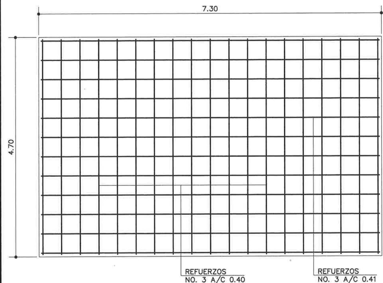
PLANTA DE LOSA
