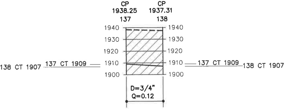
PERFIL H RED DE DISTRIBUCION 1 ESCALA HORIZONTAL 1/4000 ESCALA VERTICAL 1/8000
