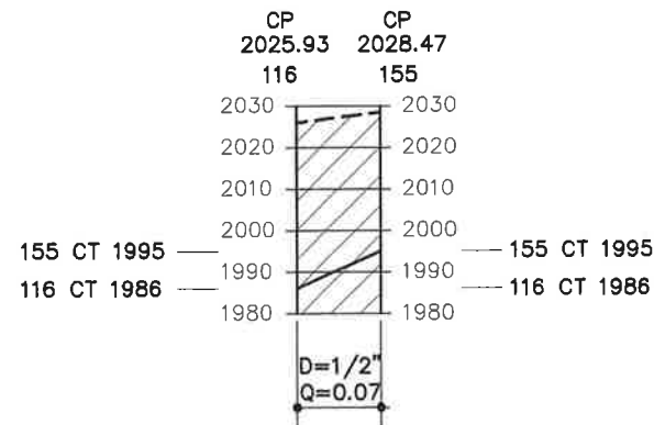
PERFIL "M" RED DE DISTRIBUCION 2 ESCALA HORIZONTAL 1/4000 ESCALA VERTICAL 1/8000
