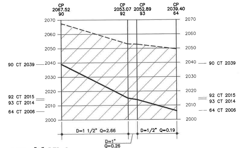
PERFIL "B" RED 2
