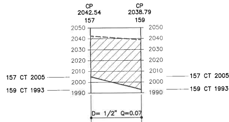
PERFIL E RED DE DISTRIBUCION 1
