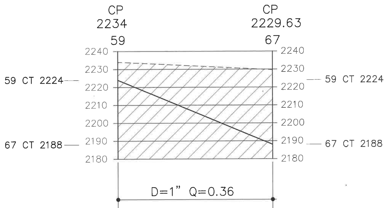
PERFIL LINEA DE CONDUCCION 59 A 67
