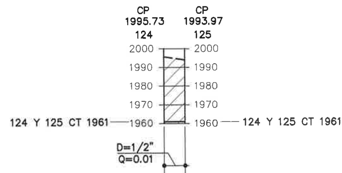
PERFIL "P" RED DE DISTRIBUCION 2 ESCALA HORIZONTAL 1/4000 ESCALA VERTICAL 1/8000
