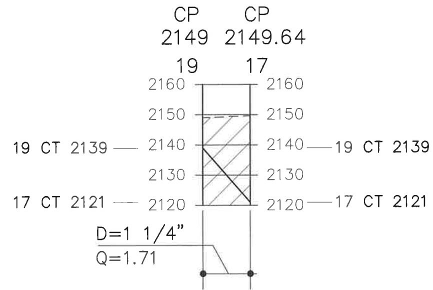
PERFIL LINEA DE CONDUCCION 19 A 17
