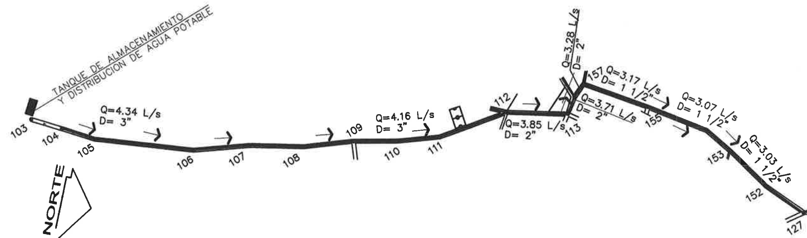
PLANTA TRAMO PERFIL A RED DE DISTRIBUCION 1
