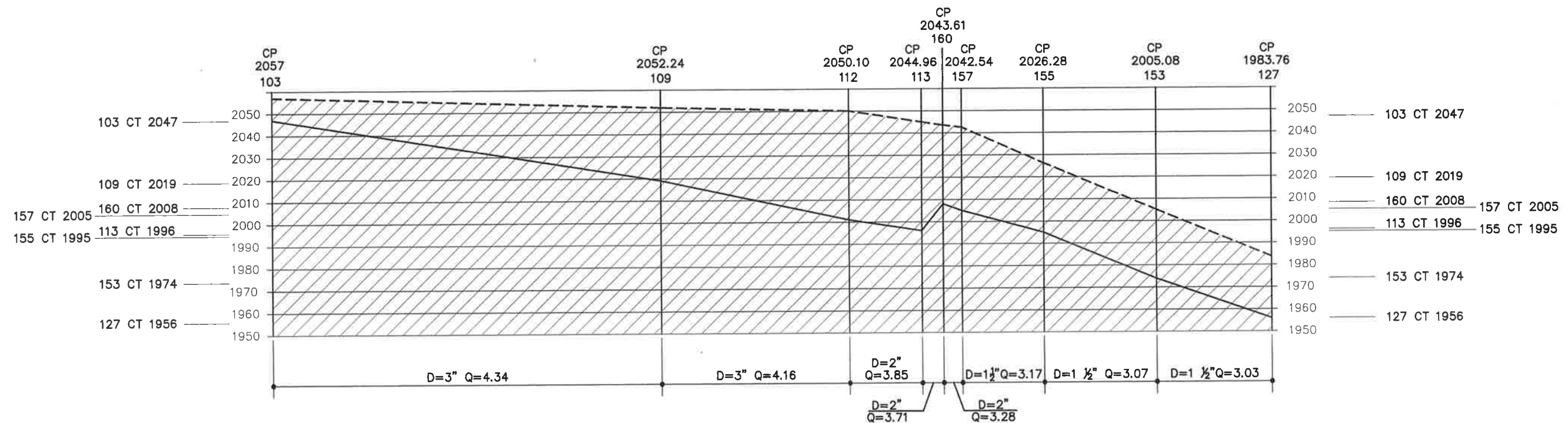
PERFIL A RED DE DISTRIBUCION 1
