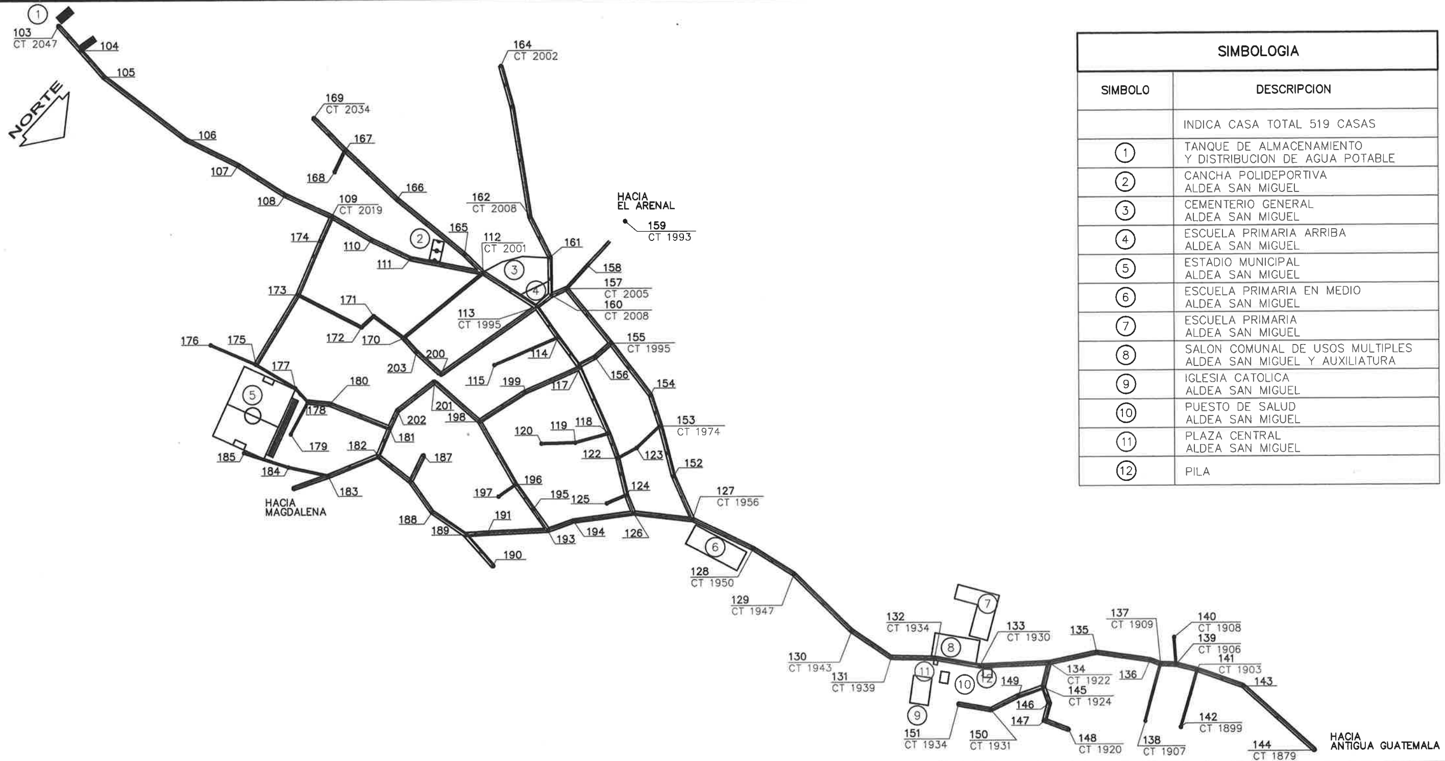
PLANTA TOPOGRAFICA ALDEA SAN MIGUEL MILPAS ALTAS SACATEPEQUEZ
