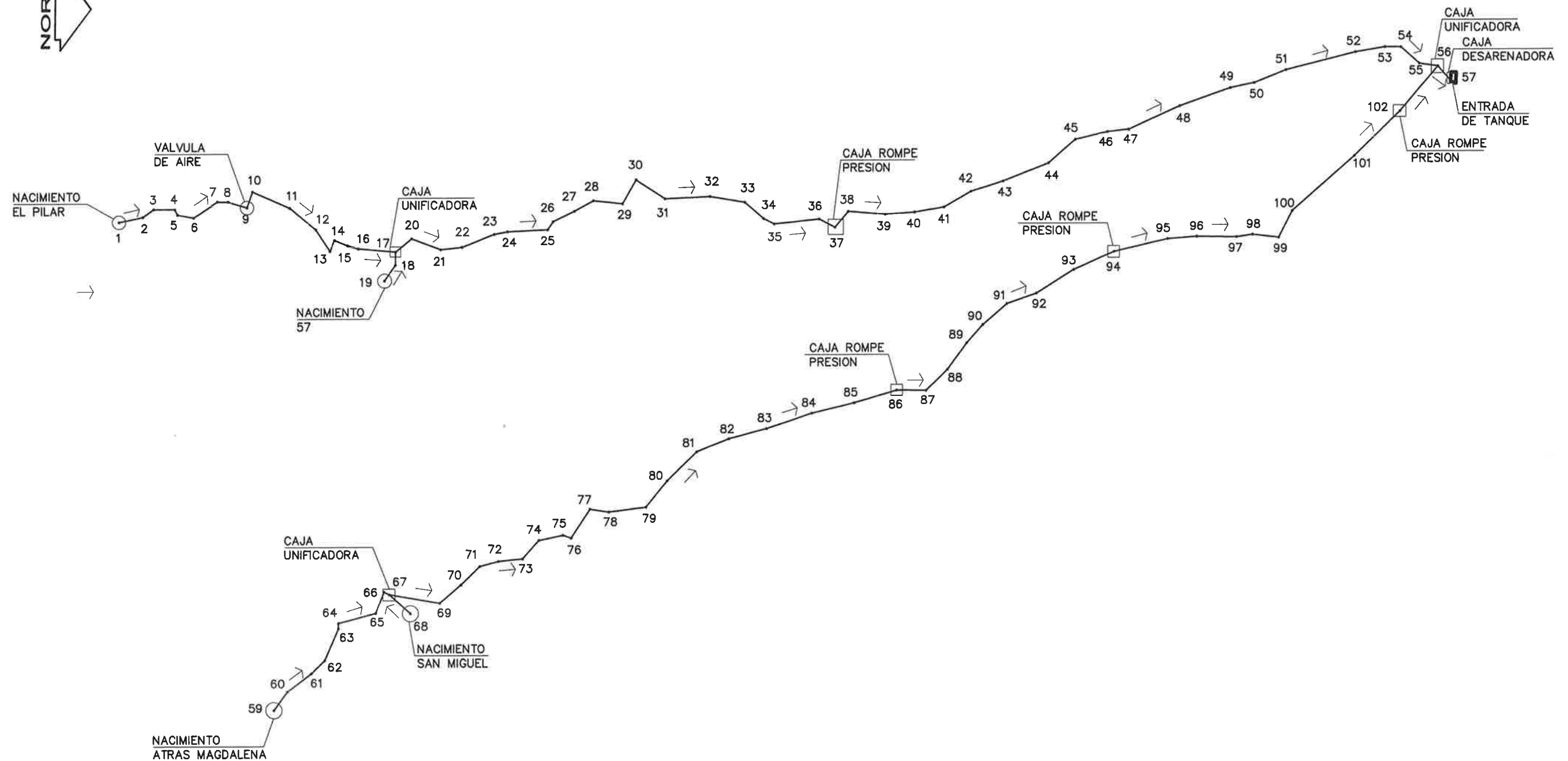
PLANTA GENERAL LINEA DE CONDUCCION ALDEA SAN MIGUEL MILPAS ALTAS SACATEPEQUEZ
