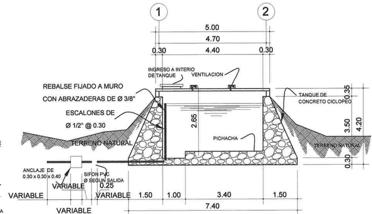
SECCION A - A' DE TANQUE DE ALMACENAMIENTO Y DITRIBUCION DE AGUA POTABLE ALDEA SAN MIGUEL
