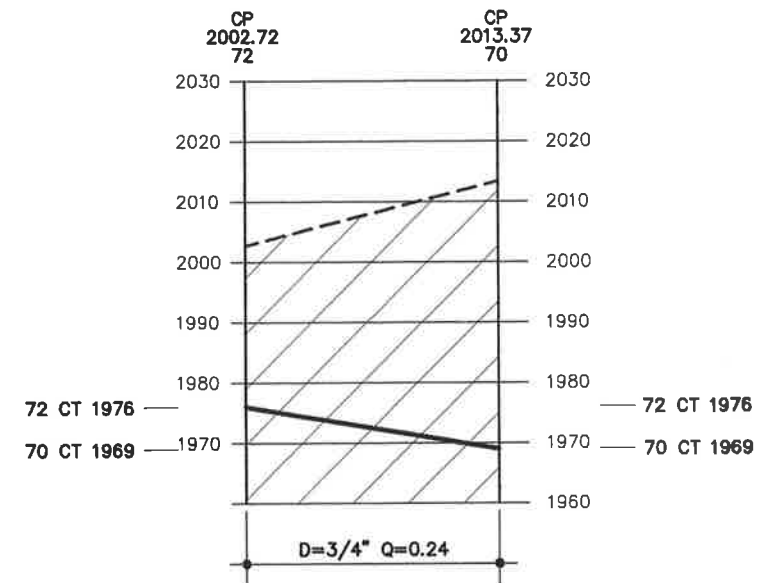
PERFIL "D" RED 1
