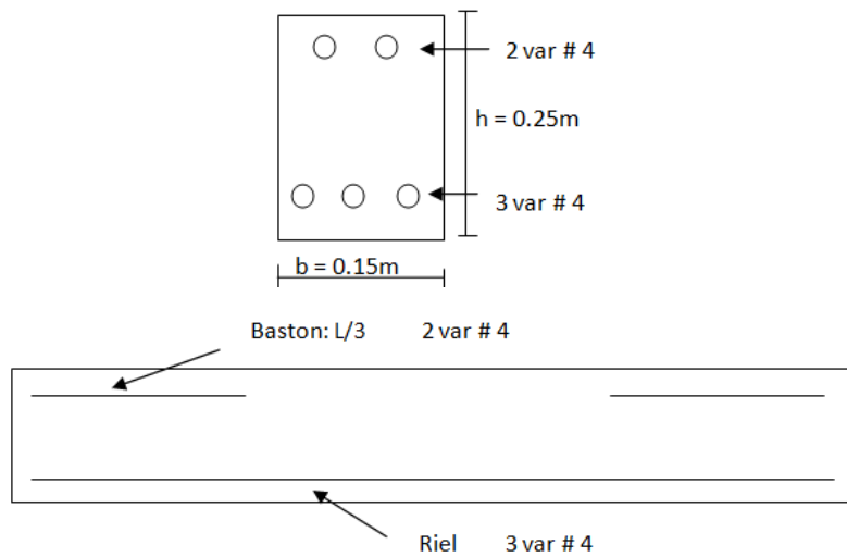
Figura 16. Refuerzo de acero viga Buena Vista
