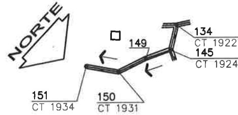
PLANTA TRAMO PERFIL F RED DE DISTRIBUCION 1 ESCALA 1/4000
