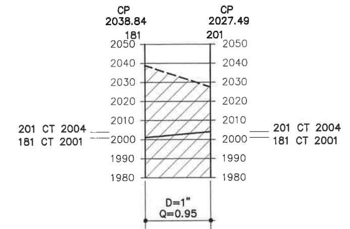
PERFIL "C'" RED DE DISTRIBUCION 2 ESCALA HORIZONTAL 1/4000 ESCALA VERTICAL 1/8000
