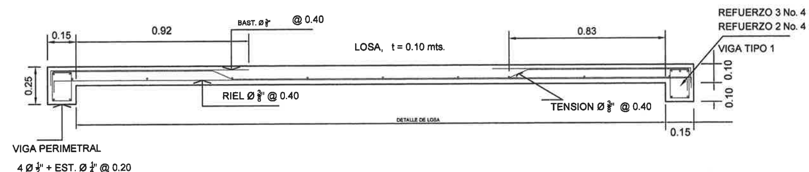
DETALLE DE LOSA
