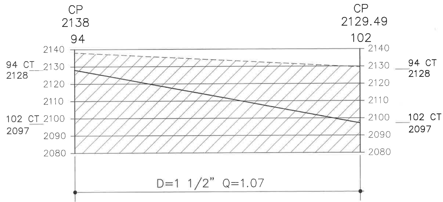
PERFIL LINEA DE CONDUCCION 94 A 102
