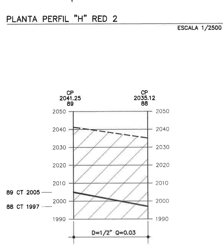
PERFIL "H" RED 2 ESCALA HORIZONTAL 1/2500 ESCALA VERTICAL 1/5000
