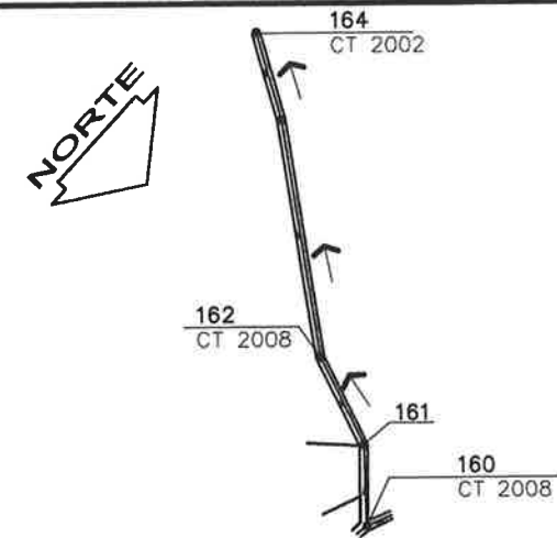
PLANTA TRAMO PERFIL D RED DE DISTRIBUCION 1
