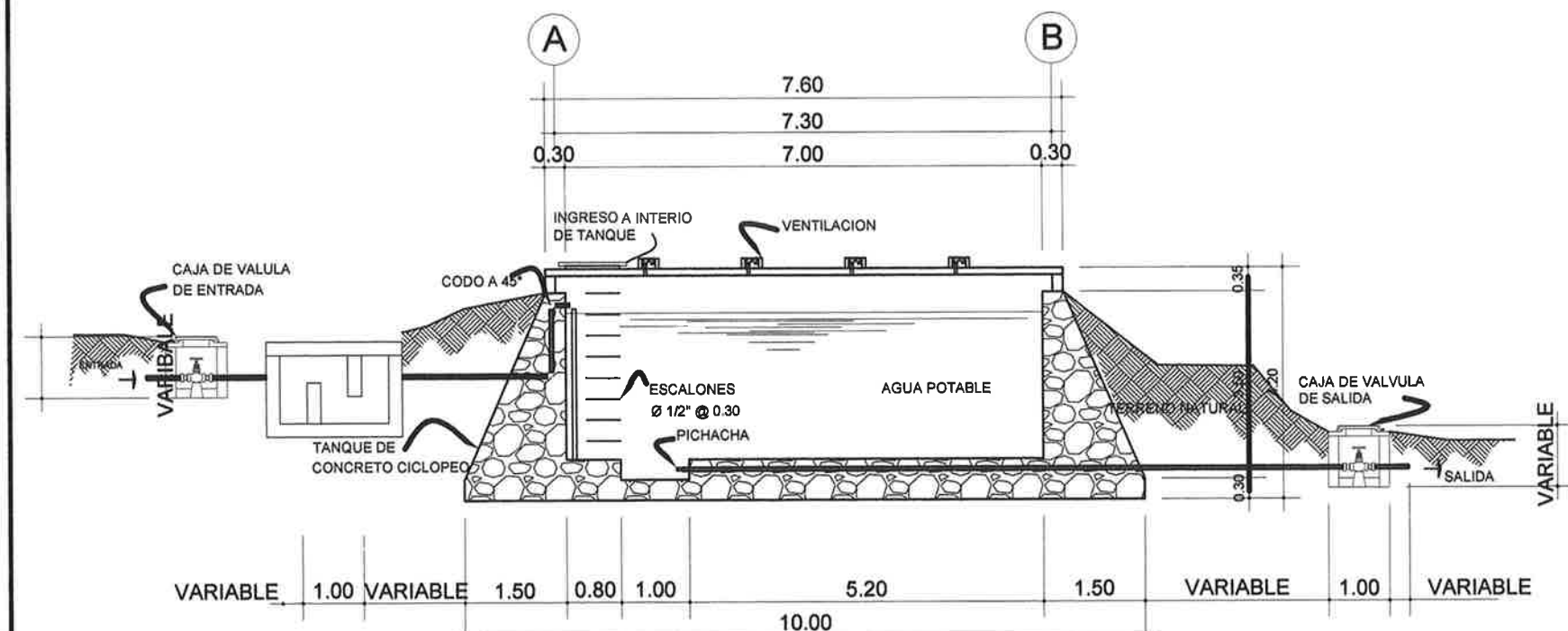
SECCION B - B' DE TANQUE DE ALMACENAMIENTO Y DITRIBUCION DE AGUA POTABLE ALDEA SAN MIGUEL
