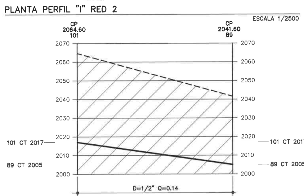
PERFIL "I" RED 2 ESCALA HORIZONTAL 1/2500 ESCALA VERTICAL 1/5000
