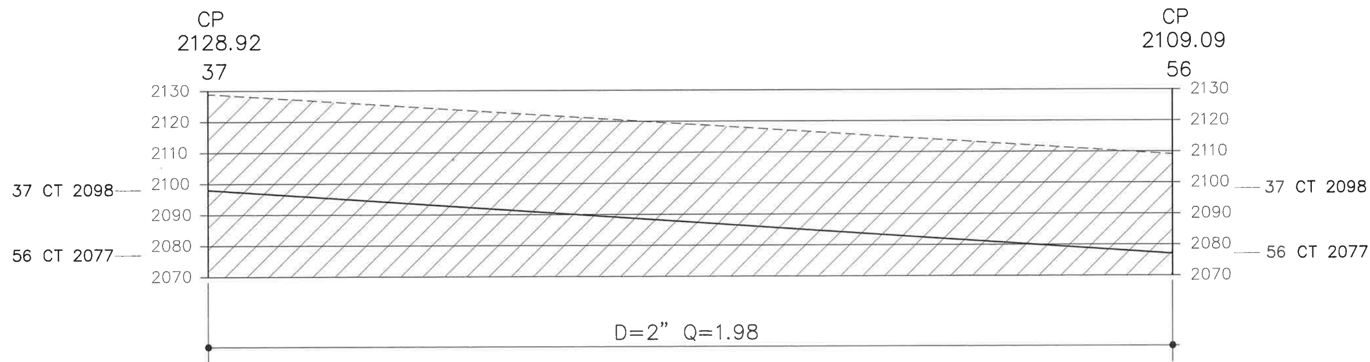
PERFIL LINEA DE CONDUCCION 37 A 56
