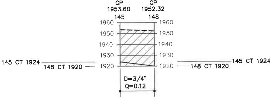
PERFIL G RED DE DISTRIBUCION 1 ESCALA HORIZONTAL 1/4000 ESCALA VERTICAL 1/8000
