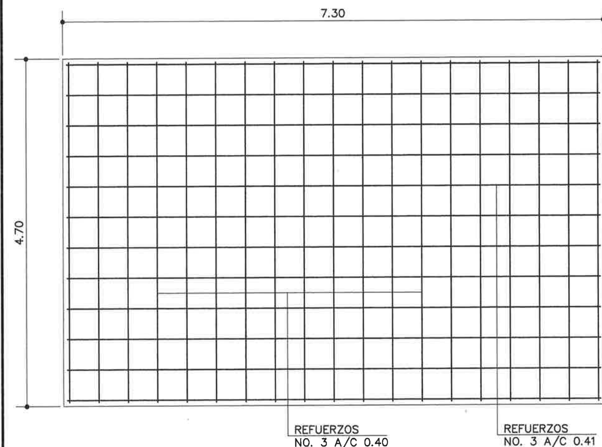
PLANTA DE LOSA
