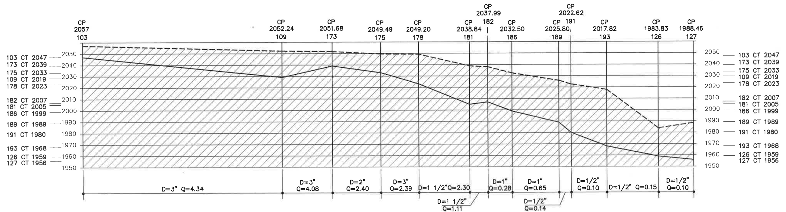
PERFIL A RED DE DISTRIBUCION 2
