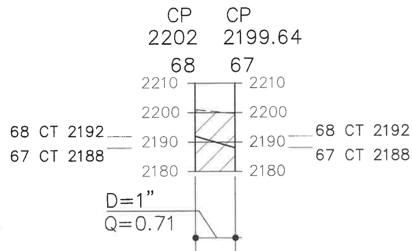
PERFIL LINEA DE CONDUCCION 68 A 67
