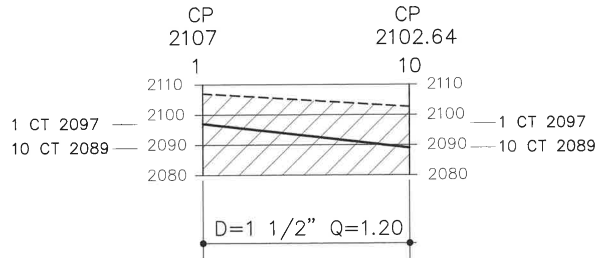
PERFIL LINEA DE CONDUCCION 1 A 10 ESCALA HORIZONTAL 1/2500 ESCALA VERTICAL 1/5000
