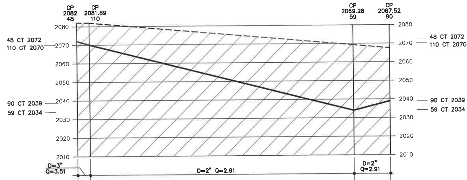
PERFIL "A" RED 2
