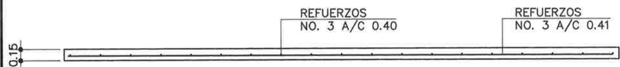
SECCION DE LOSA
