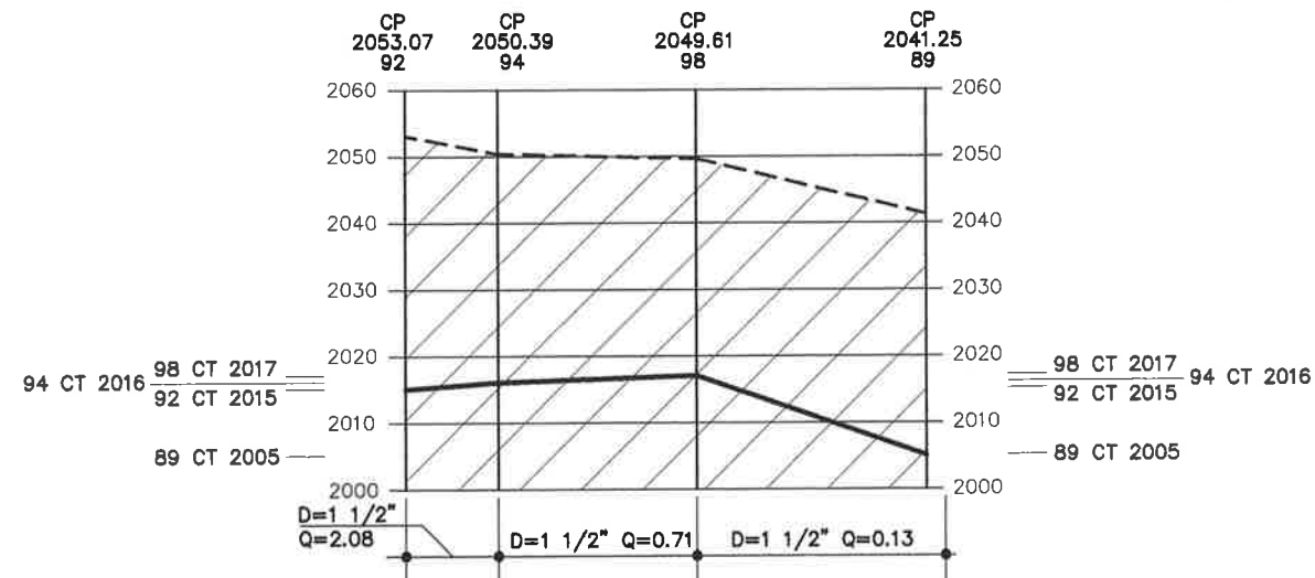
PERFIL "C" RED 2
