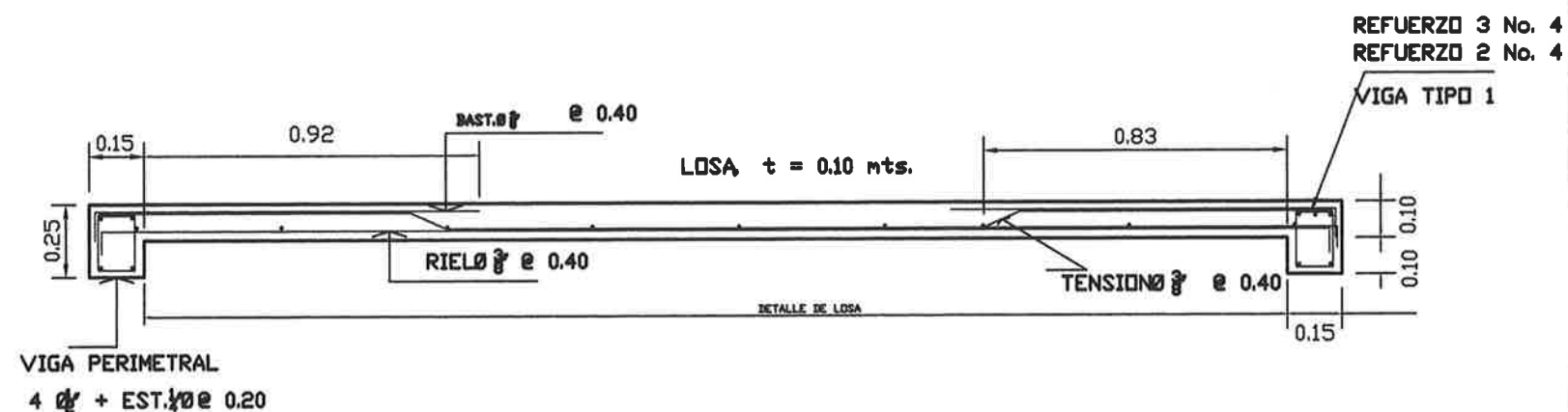
DETALLE DE LOSA
