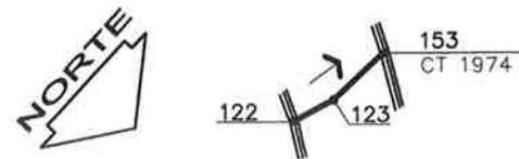
PLANTA TRAMO PERFIL "O" RED DE DISTRIBUCION 2 ESCALA 1/4000
