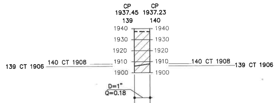
PERFIL I RED DE DISTRIBUCION 1
