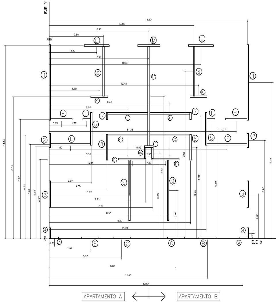
Figura 26. Medida de centroide de muros
