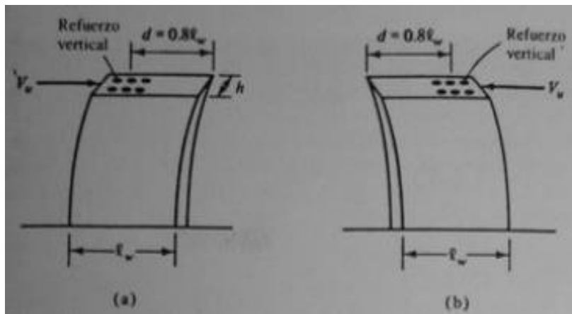
Figura 35. Muros de cortante
