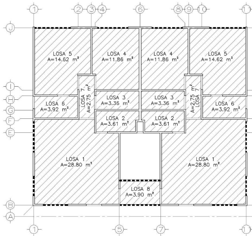
Figura 23. Área de losas
