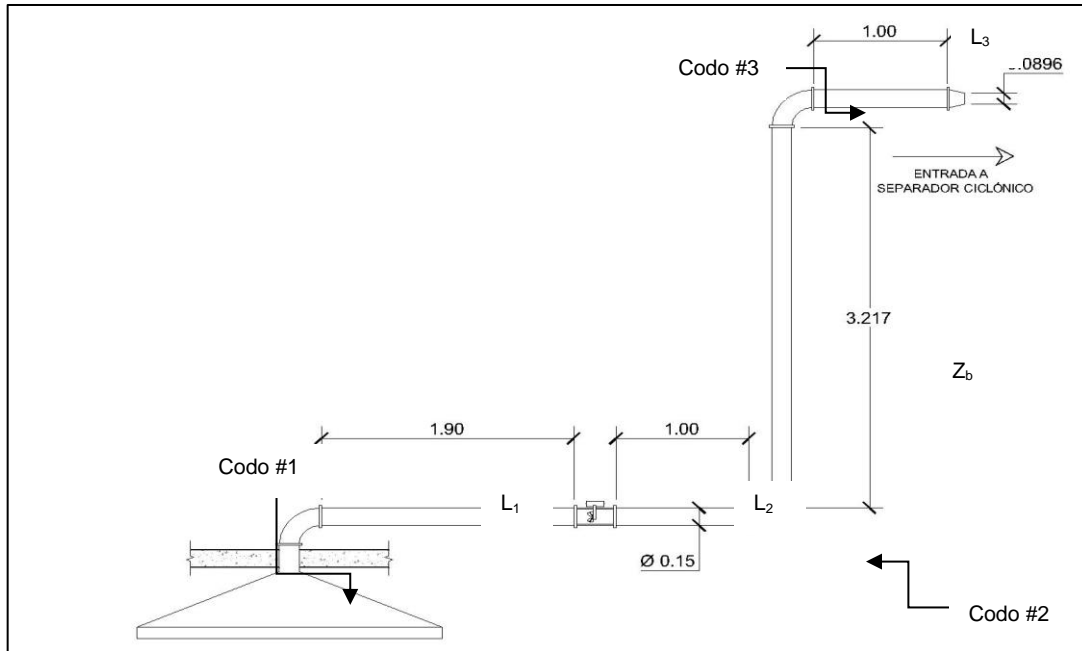
Figura 8. Sistema de ductos de carga y descarga al sistema de extracción propuesto
