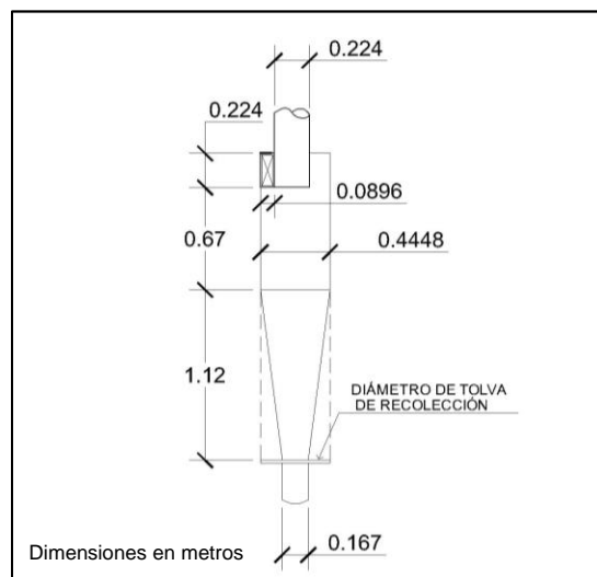
Figura 15. Separador ciclónico de alta eficiencia Stairmand
