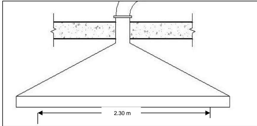
Figura 7. Diámetro de campana de extracción suspendida
