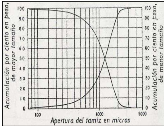
Figura 3. Acumulación de tamaños-distribución
