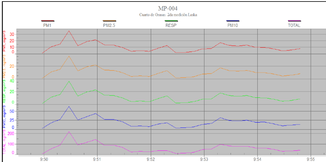
Figura 14. Concentración de partículas de almidón en polvo en función del tiempo para un diámetro de partícula dado
