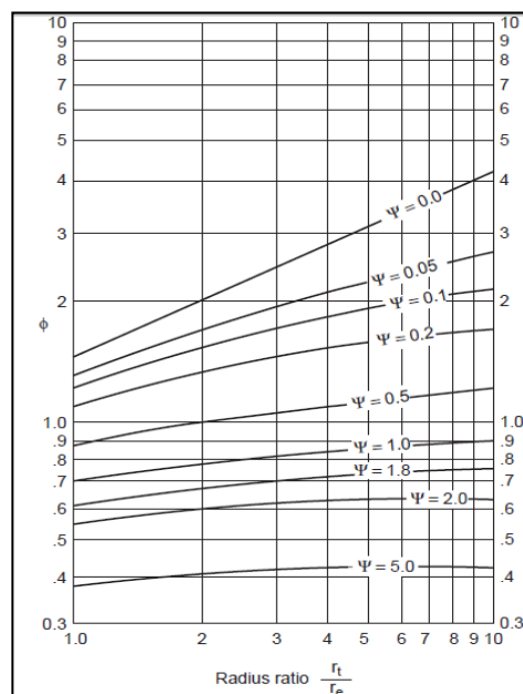
Figura 12. Factor de caída de presión del ciclón
