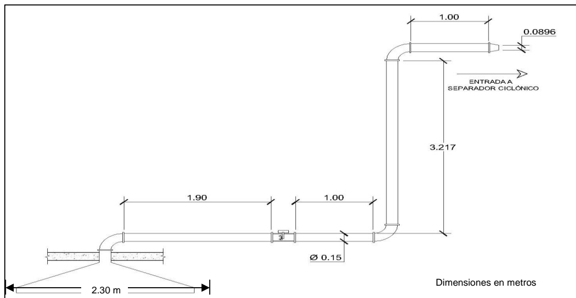
Figura 17. Sistema de ducto de carga y descarga al separador ciclónico
