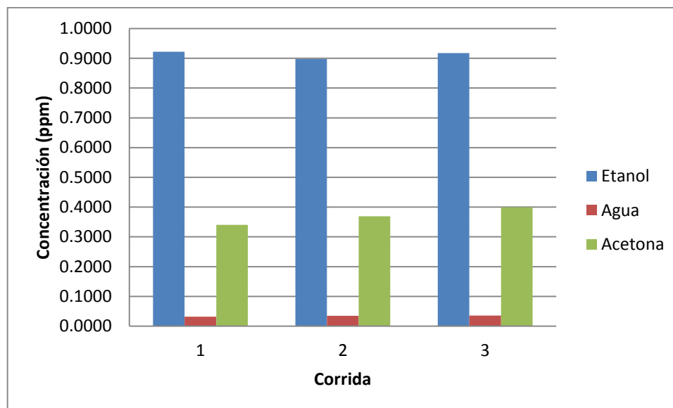
Figura 6. Concentración de \beta -caroteno obtenido del extracto de la cáscara de banano en función del solvente utilizado
