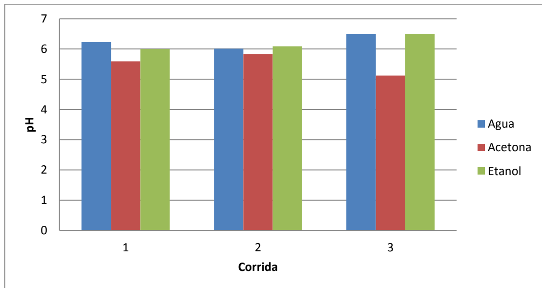
Figura 8. Potencial de hidrógeno del extracto de \beta -caroteno sin concentrar obtenido de la cáscara de banano
