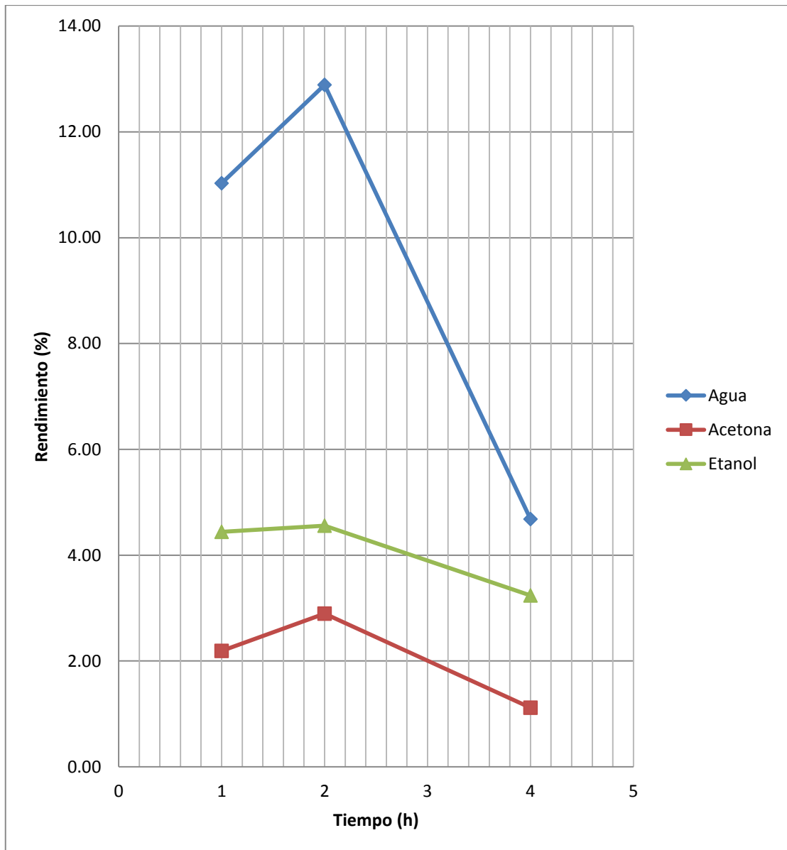
Figura 4. Evaluación del tiempo de extracción de \beta -caroteno obtenido de la cáscara de banano utilizando tres solventes, para fijar la variable del tiempo de extracción
