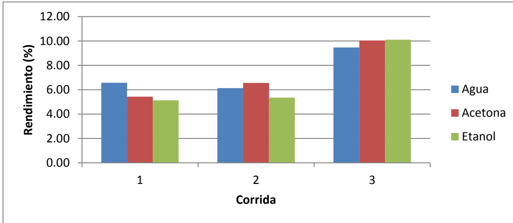
Figura 5. Rendimiento del extracto de \beta -caroteno obtenido de la cáscara de banano en función del solvente utilizado
